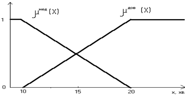
Рисунок.А.2 - Функції приналежності \mu^{\text{дов}}(x) та \mu^{\text{нед}}(x)
