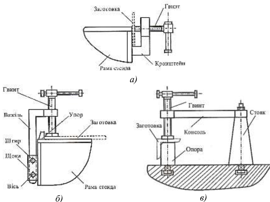
а – постійний, б – відкидний, в – поворотний Рисунок 2.1 – Гвинтові притискачі [1]
