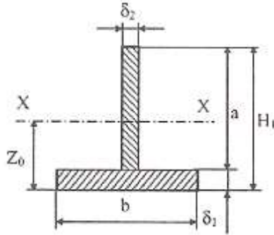
Рисунок 2.4 – Схема розрахунку поперечного перерізу корпусу гвинтового притискача
