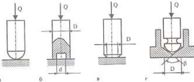
Рисунок 2.3 – Види контакту гвинта з опорною поверхнею [1]
