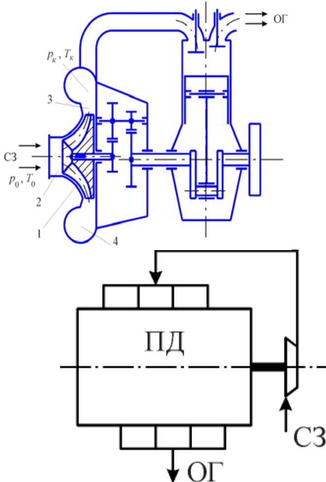
Рис. 1. Принципова схема комбінованого двигуна з механічним способом наддуву
