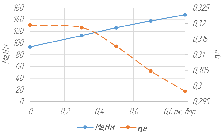
Рисунок 7.2 – Ефективний крутний момент та ефективний ККД двигуна, при різних значеннях тиску наддуву
