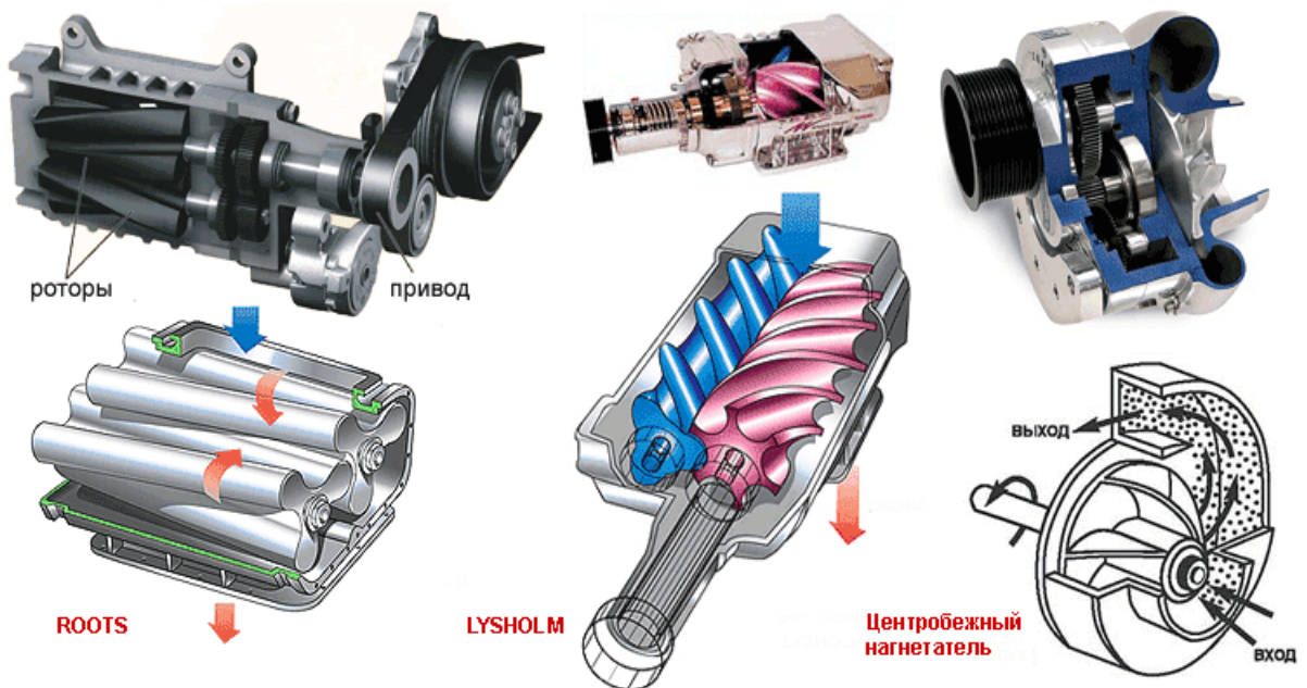
Рисунок. – Механічні нагнітачі.
