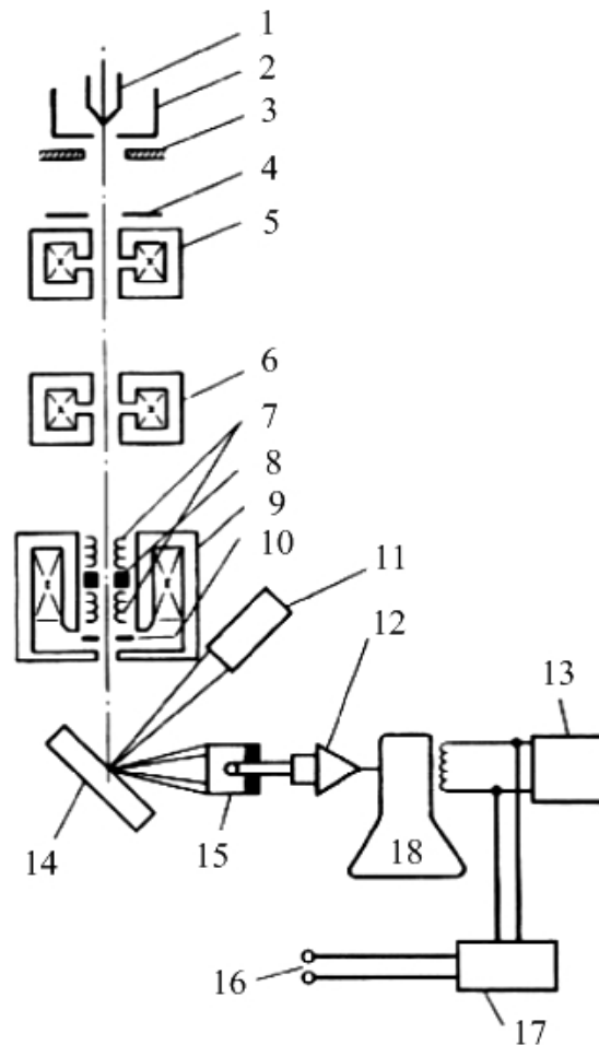
Рисунок 2.4 – Схема електронної оптики РЭММА:
