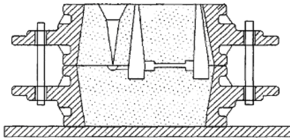
Рисунок 2.1 – Схема ливарної форми для одержання зразків
