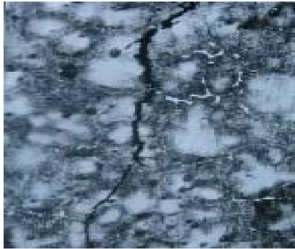
Рисунок 3.3 – Розповсюдження тріщини в сплаві МЛ5 по межах зерна, х200
