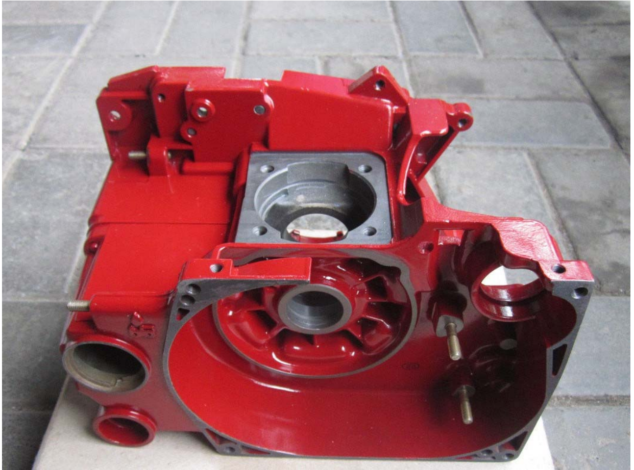
Рисунок 3.1 – Корпус картера зі сплаву МЛ5
