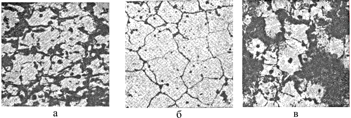
Рисунок 1.8 – Мікроструктура сплаву МЛ5, \times 100 : а – в литому стані; б – в загартованому стані ; в – після гартування і старіння [5]
