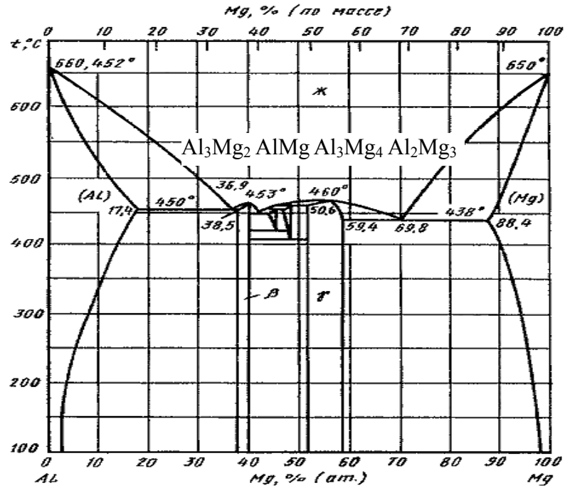
Рисунок 1.3 – Mg–Al Діаграма стану [7]
