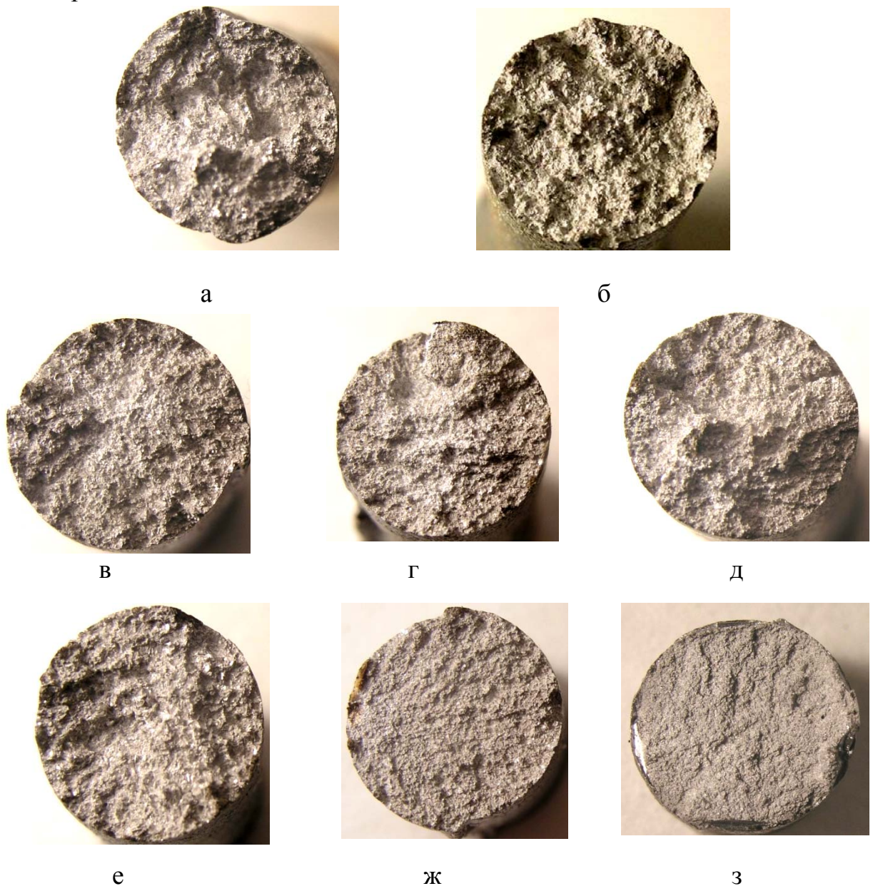
Рисунок – 3.4 Злами зразків зі сплаву МЛ5 з Ca и Ba, х5: а – без модифікування; б – 0,05 % Ca; в – 0,1 % Ca; г – 1,0 % Ca;
