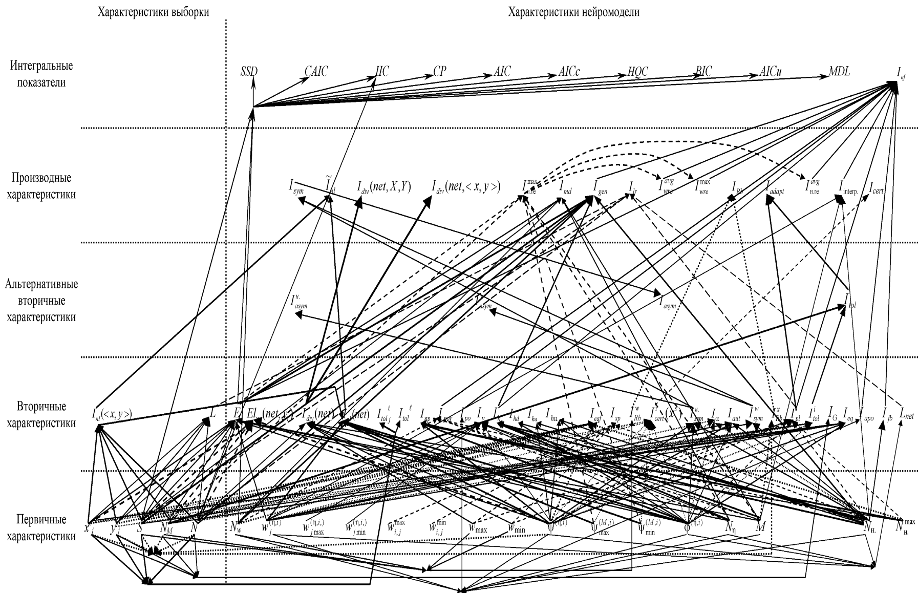
Рис. 1. Схема аналитических взаимосвязей информационных показателей качества диагностических нейромоделей
