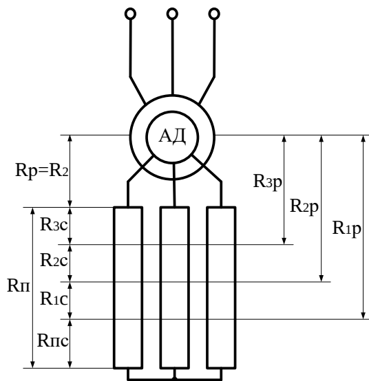
Рисунок 1.8 – Принципова схема силової частини електропривода змінного струму
