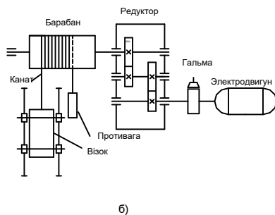
Рисунок 1.1 – Кінематична схема похилого підйомника
