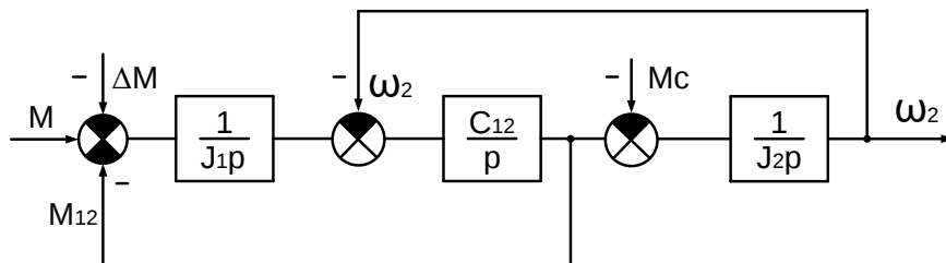
Рисунок 1.3 - Структурна схема
