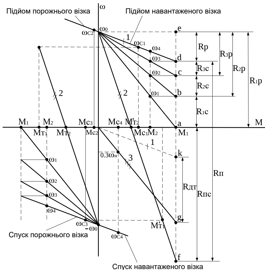
Рисунок 1.6 – Діаграми пускова і гальмівна
