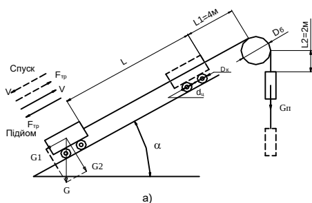
Рисунок 1.1 – Кінематична схема похилого підйомника
