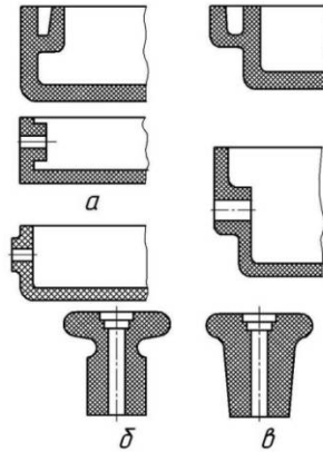
Рисунок 2.11 - Приклади усунення зовнішніх і внутрішніх піднутрinių
