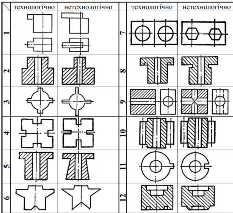
Рисунок 3.2. - Приклади конструкції порошкових виробів
