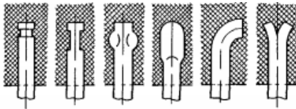
Рисунок 2.15 - Варіанти закріплення дротяної арматури
