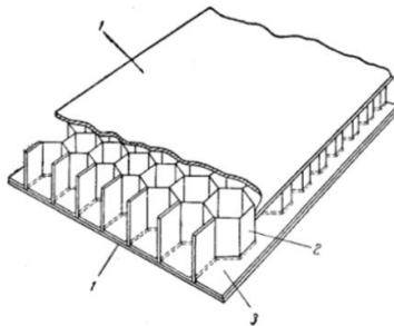
Рисунок 2.17 - Панель сотової конструкції
