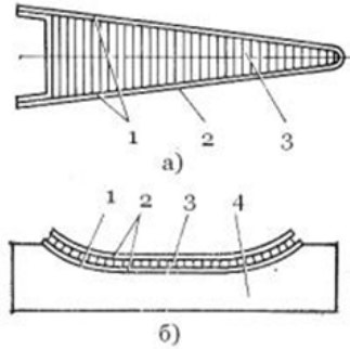
1 – базова поверхня; 2 – обшивка; 3 – заповнювач; 4- шаблон Рисунок 2.18 - Формування виробу по стільниковому заповнювачу (а) і по шаблону (б)
