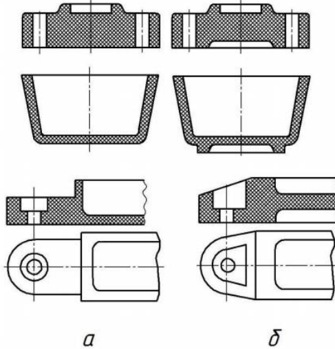
а – нетехнологічно; б – технологічно Рисунок 2.10 - Приклади оформлення заглиблень і опорних поверхонь
