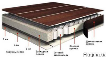
Рисунок 2.19 - Приклад використання закладної планки і декоративної стрічки
