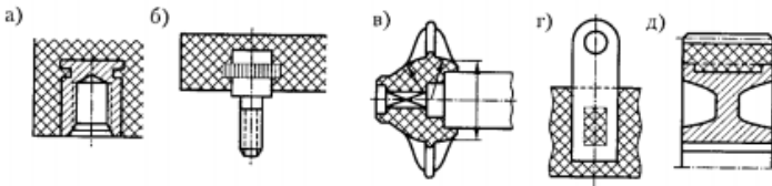
а – втулкова; б – стрижнева рифлена; в – стрижнева квадратна; г – плоска; д – кільцева
