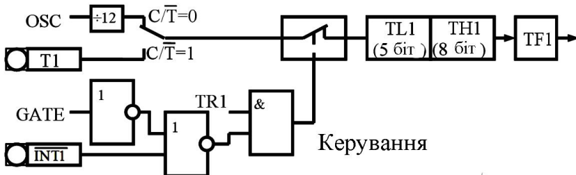
Рисунок 5.1 – Структура таймера/лічильника в режимі 0
