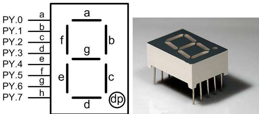
Рисунок 2.1 - Семисегментний індикатор
