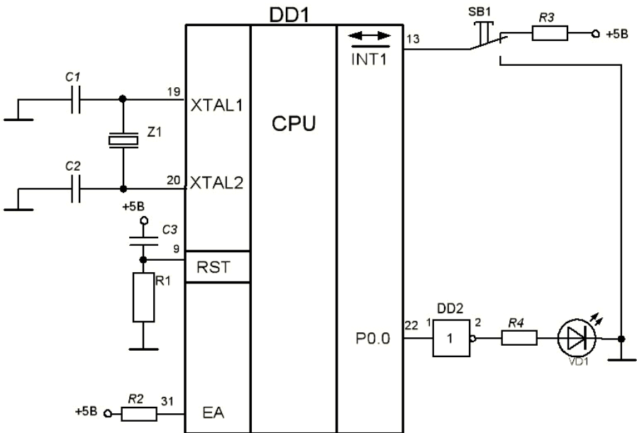
Рисунок 5.3 – Схема з'єднання МК з органами керування та світлодіодом
