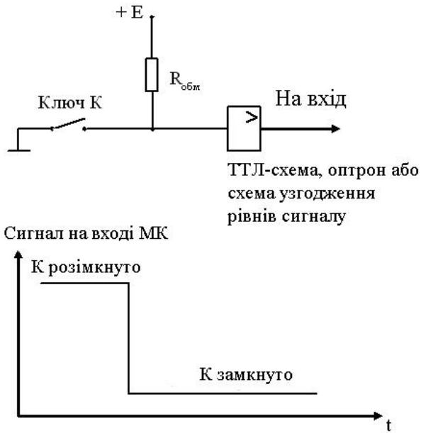
Рисунок 3.1 - Схема двійкового давача
