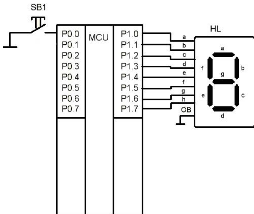
Рисунок 3.4 – Апаратна частина завдання
