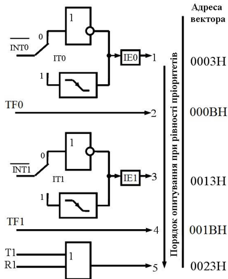
Рисунок 4.1 - Система переривань МК-51
