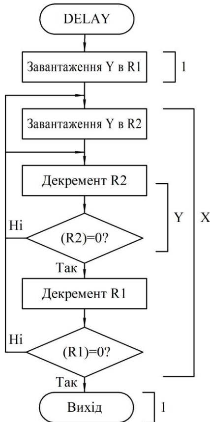
Рисунок 3.3 - Структурно-алгоритмічна схема формування часової затримки
