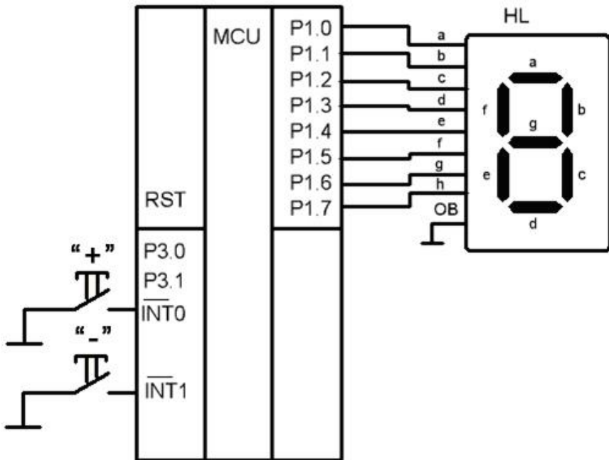
Рисунок 4.2 – Схема з'єднання МК з органами керування та індикатором
