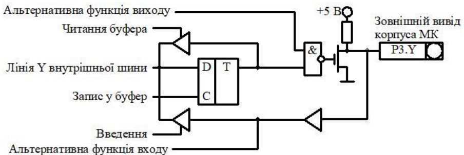
Рисунок 3.1 - Спрощена принципова схема порту 3
