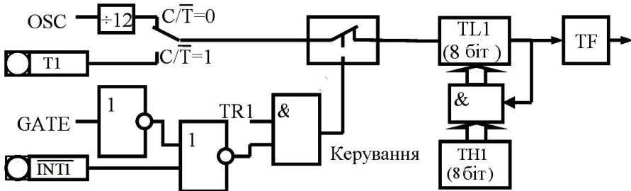
Рисунок 5.2 – Структура таймера / лічильника в режимі 2
