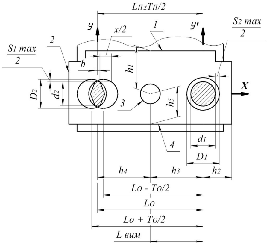
Рисунок 1.4 – Установка на циліндричний и зрізаний пальці
