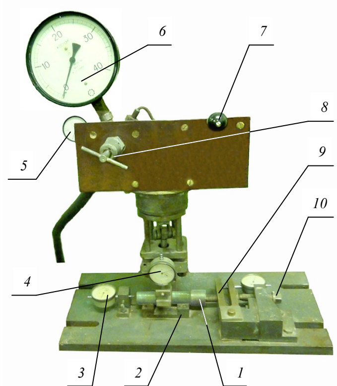
Рисунок 4.2 – Експериментальний стенд
