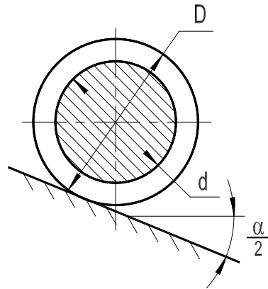
Рисунок 6.3 – Клиновий механізм
