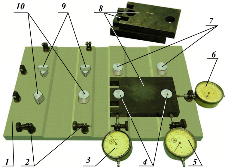
Рисунок 1.5 – Експериментальний стенд
