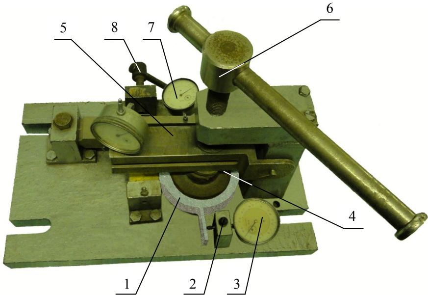
Рисунок 3.2 – Експериментальний стенд
