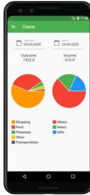
Рисунок 4 – Сторінка статистики
