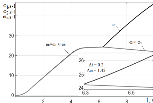
Рисунок 14. Швидкості двох коліс і приведена до ЕМБ кутова швидкість
