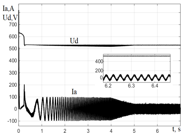
Рисунок 13. Напруга живлення та струм фази А
