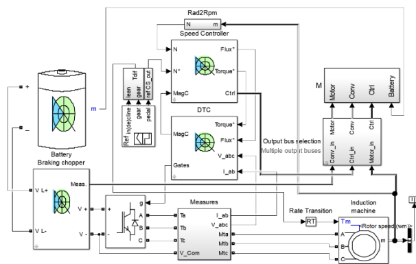
Рисунок 3. Імітаційна модель ЕП
