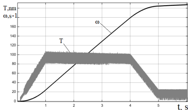
Рисунок 8. Швидкість і момент двигуна при пуску без пробуксовки
