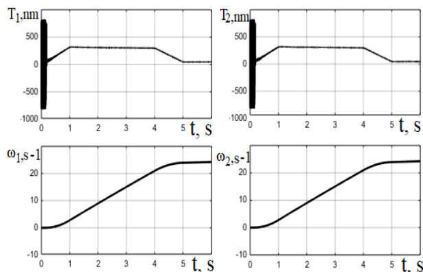
Рисунок 9. Швидкості та крутні моменти дво коліс при руханні без пробуксовки
