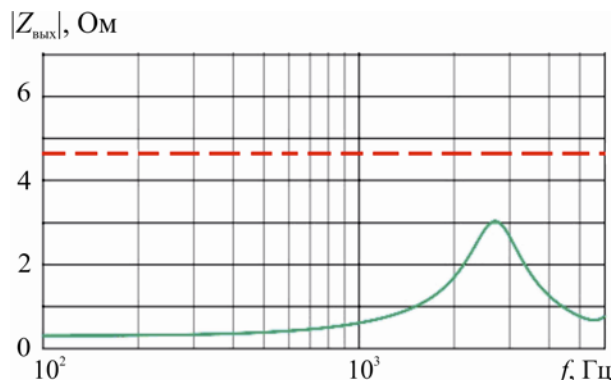
Рисунок 12. Частотные зависимости выходного сопротивления сетевого фильтра радиопомех и входного сопротивления ИПН (-----), показывающие выполнение условия Z_{\text{вых}}^{(1)}(j\omega)/Z_{\text{вх}}^{(2)}(j\omega) \neq -1 .
