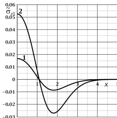
Рисунок 5. Розподіли нормальних напружень в точках одностарової основи:
