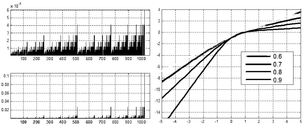
Рис. 1. Реализации каскада (а) и скейлинговые экспоненты \tau(q) для разных p_1 (б)
