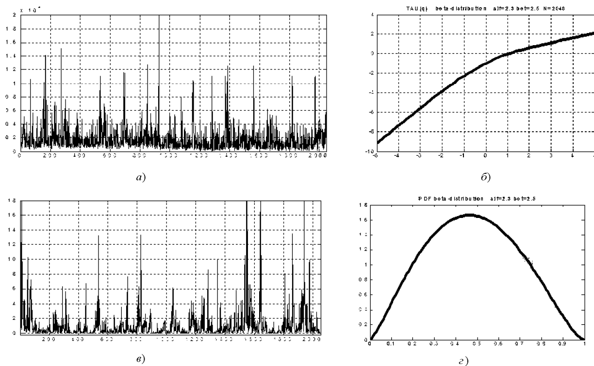
Рис. 5. Реализация трафика (а), выборочная скейлинговая экспонента \tau(q) (б), плотность бета-распределения a=2.3, b=2.5 (г), модельная реализация (в)
