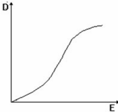
Рисунок 2.3 – Типовий графік залежності електричної індукції від напруженості поля D = f(E)
