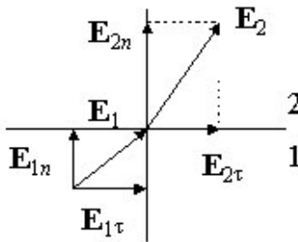
Рисунок 5.3 – Переломлення ліній електричного поля
