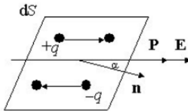
Рисунок 3.1 – Поляризація діелектрика
