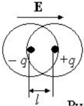
Рисунок 2.1 – Зміщення зарядів всередині молекули у зовнішньому електричному полі
