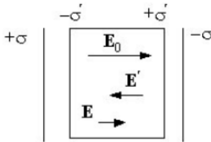
Рисунок 3.2 – Плоский однорідний діелектричний шар між двома різнойменно заря-
