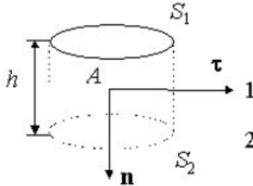
Рисунок 5.1 – Поверхня діелектрика у вигляді циліндра
