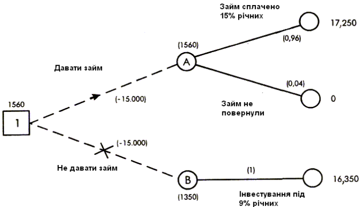
Рисунок 1.1 – Дерево рішень
