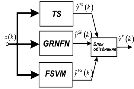
Рис. 2. Ансамбль нейро-фаззі систем
