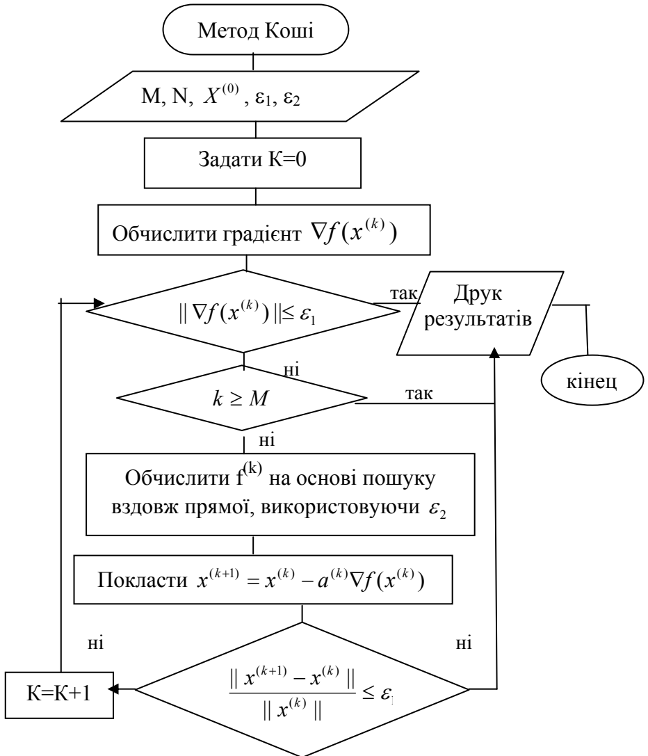
Рисунок 1.1 – Схема методу Коші
