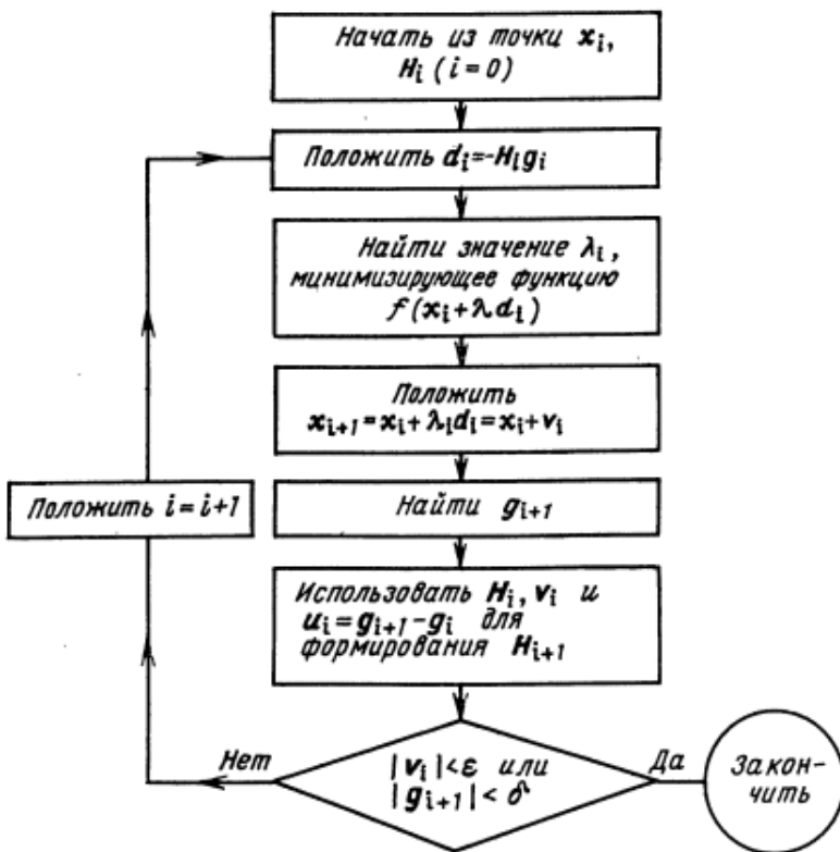
Рисунок 5.1 - Спрощена блок-схема алгоритму Девідона-Флетчера-Пауелла.
