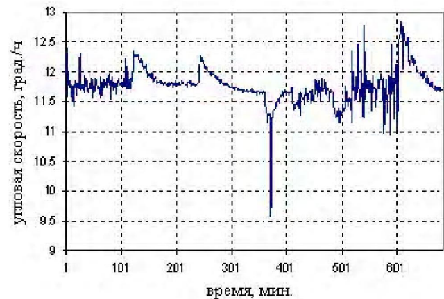
Рис. 5. Аппроксимация экспериментальных измерений моделью (2)
