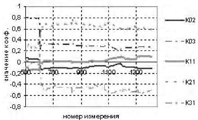
Рис. 4. Динамика оценок параметров модели (2)
