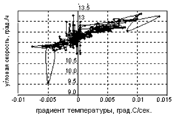
Рис. 2. Зависимость измерений угловой скорости от градиента температуры
