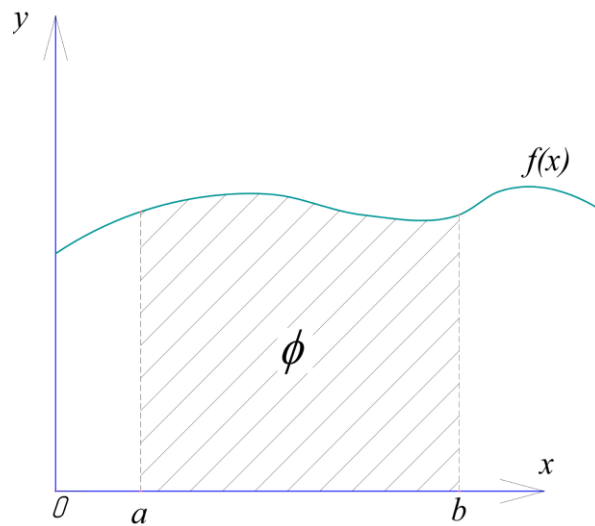
Рис. 1. Графічна інтерпретація фізичного змісту функціоналу виду (9)
