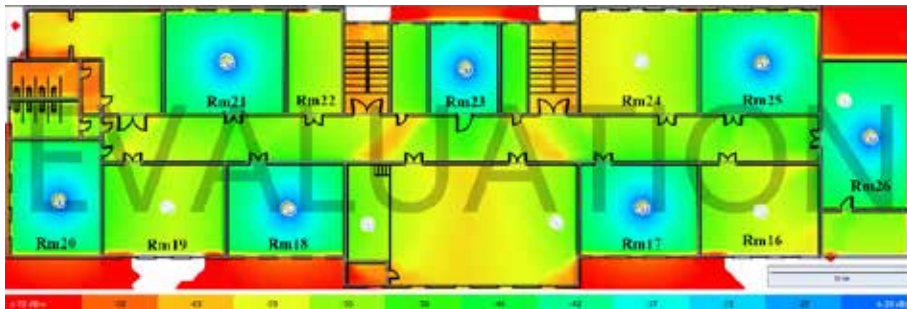
Рис. 4. Рівень сигналу на другому поверсі в діапазоні 5 ГГц
