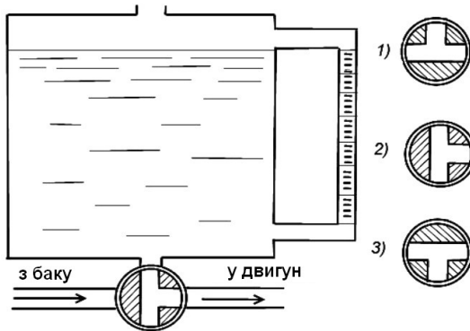
Рисунок 6.8 – Схема побудови мірного циліндру
