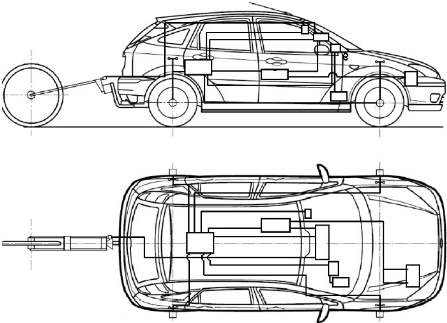
Рисунок 6.4 – Установлене "п'ять колесо" фірми Peiseler на Ford Focus та схема розміщення вимірювальної апаратури на автомобілі
