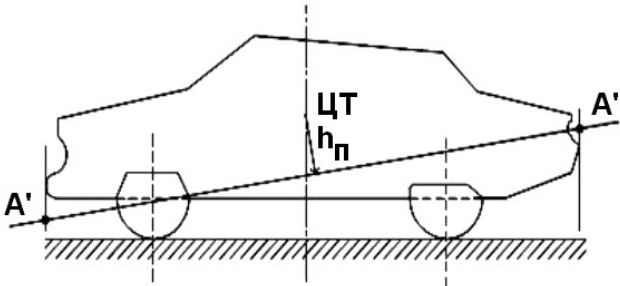
Рисунок 7.4 - Розташування осі поперечних коливань
