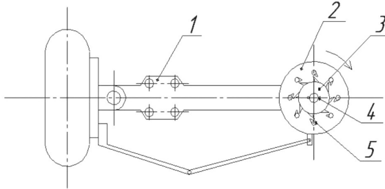
1 - передня вісь; 2 - поворотний диск; 3 - храпове колесо; 4 - контакти; 5 - храповик
