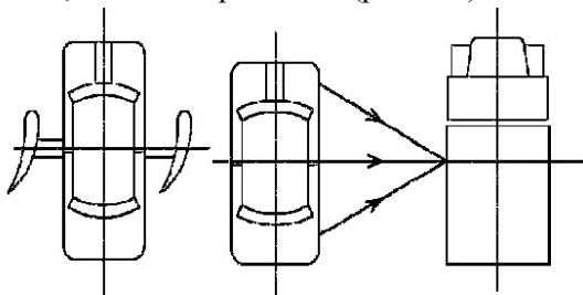
Рисунок 7.9 - Схеми створення бічної сили
