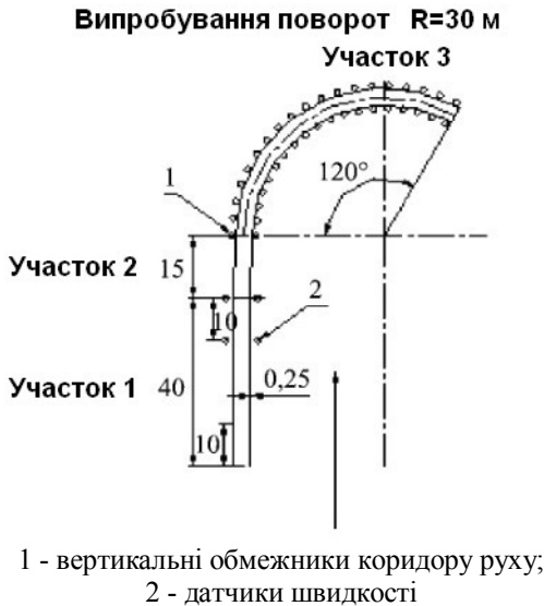
Рисунок 7.19 - Випробування "поворот" з радіусом 30 м:
