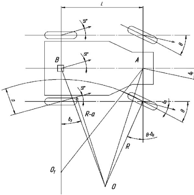
Рисунок 7.8 - Схема уводу автомобіля на повороті
