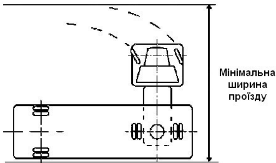
Рисунок 7.24 - Ширина проїзду автопоїзда
