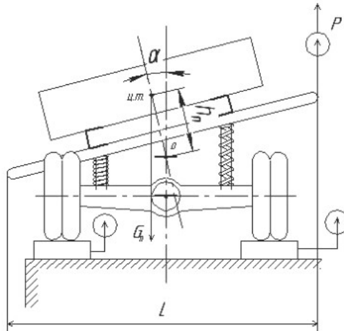
Рисунок 7.3 - Схема визначення кутової твердості підвіски автомобіля
