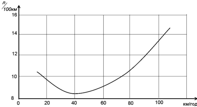
Рисунок 6.11 - Вид дорожньої економічної характеристики автомобіля
