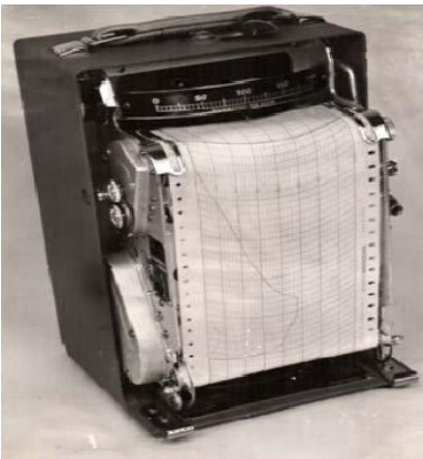
Рисунок 6.5 – Прилад реєстрації "п'ятого колеса"
