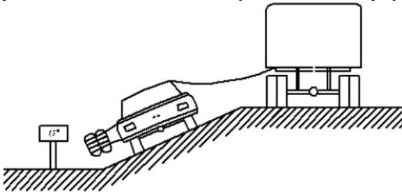
Рисунок 7.1 - Схема випробувань на косоугорі
