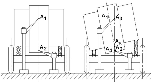
Рисунок 7.5 - Схема визначення осі поперечних коливань
