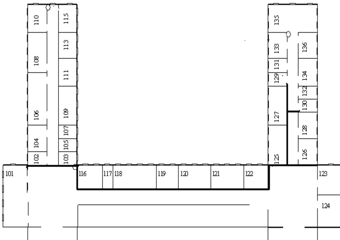
Рисунок Б.5 - Карта – схема прокладки дровових трас приміщення №1
