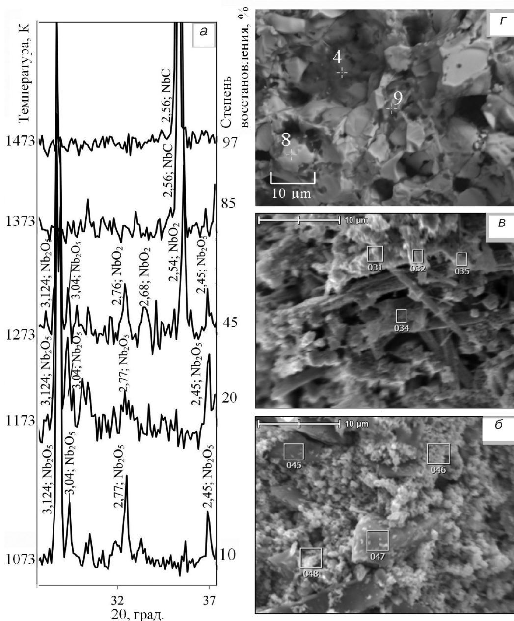
Рис. 2. Участок дифрактограмм (а) и фрактограммы ниобийсодержащих таблеток на основе Nb 2 O 5 с содержанием 15 %мас. флюса АН-295 после углеродотермического восстановления с увеличением \times 4000 (б-в), \times 2000 (г), восстановленных при температурах, К: б – 1073; в – 1273; г – 1473
