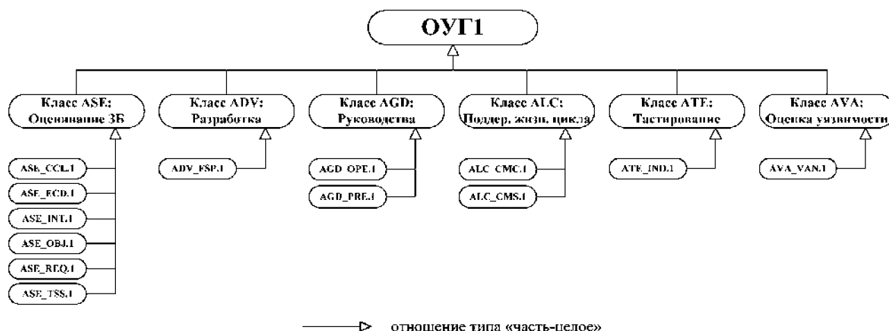
Рис. 3. Иерархическая объектно-ориентированная онтология требования гарантий по ОУГ1
