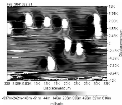
Рис. 6. Карта розподілу локальних корозійних струмів в умовах інтенсивного пітингоутворення на циклічно деформованій поверхні сталі 08X18H12T у середовищі pH6,5
