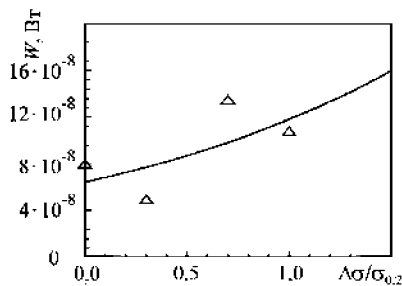
Рис. 4. Залежність параметра W від відношення \Delta\sigma/\sigma_{0,2}
