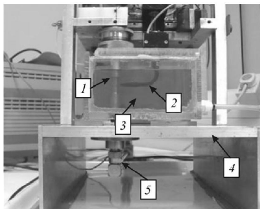
Рис. 1. Загальний вигляд установки для електрохімічного сканування циклічно деформованої поверхні за методикою SRET [11, 12]
