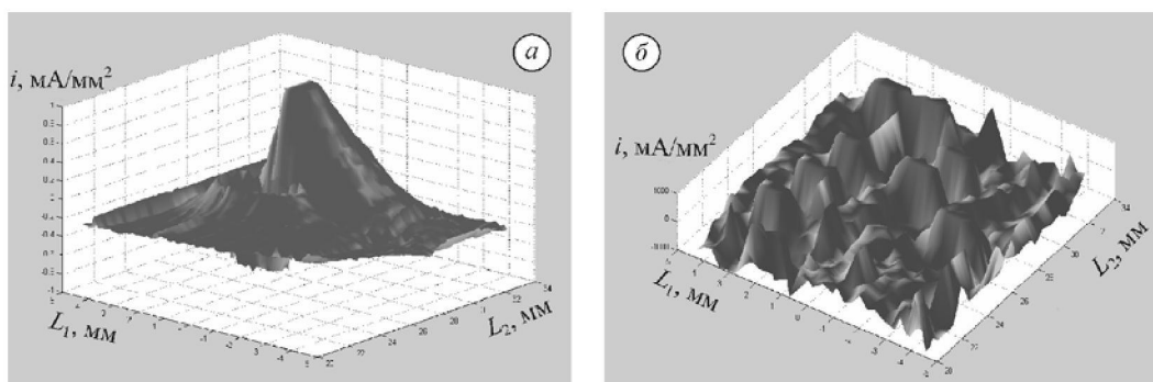
Рис. 7. Трьохмірний розподіл локальних корозійних струмів для випадку поодинокого пітингу (а) та інтенсивного пітингоутворення (б) на циклічно деформованій поверхні сталі 08X18H12T у середовищі pH6,5
