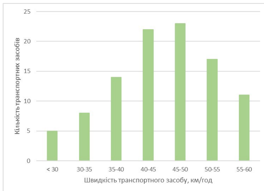
Рисунок 1.22 - Швидкості руху автомобілів Дніпровським шосе з боку вулиці Дудикіна
