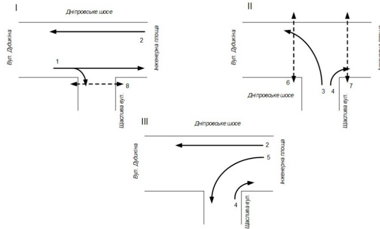
Рисунок 1.7 – Діючі фази регулювання
