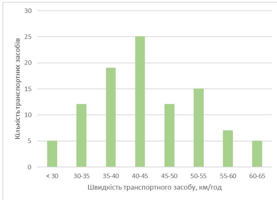
Рисунок 1.21 - Швидкості руху автомобілів Дніпровським шосе з боку вулиці Бориспільської
