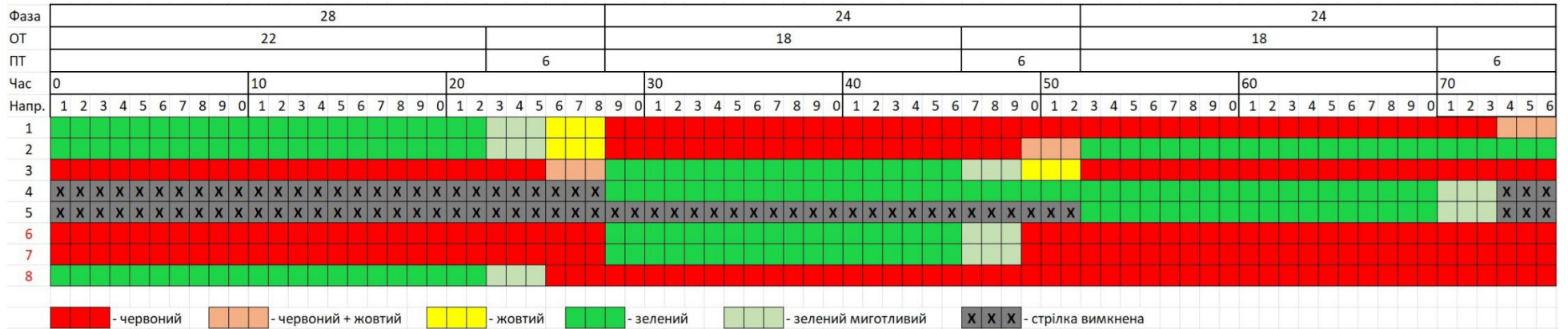
Рисунок 2.4 - Циклограма роботи світлофорів за програмою III
