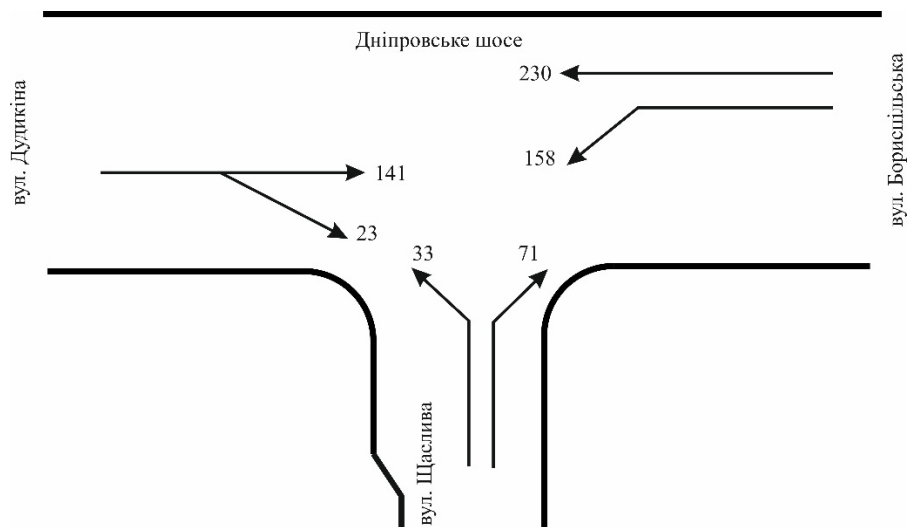
Рисунок 1.18 – Приведені об’єми руху (з 13:00 до 14:00)
