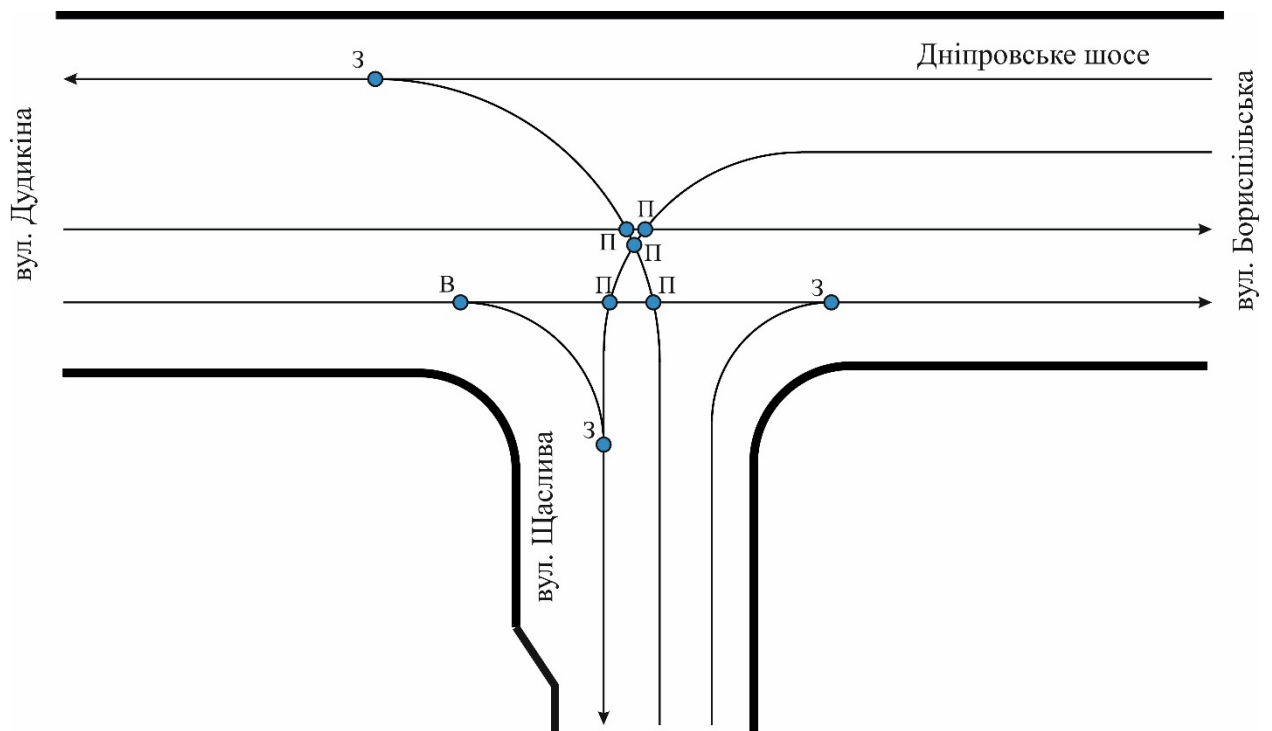
Рисунок 1.11 – Наявні конфліктні точки на перехресті Дніпровського шосе із вулицею Щасливою
