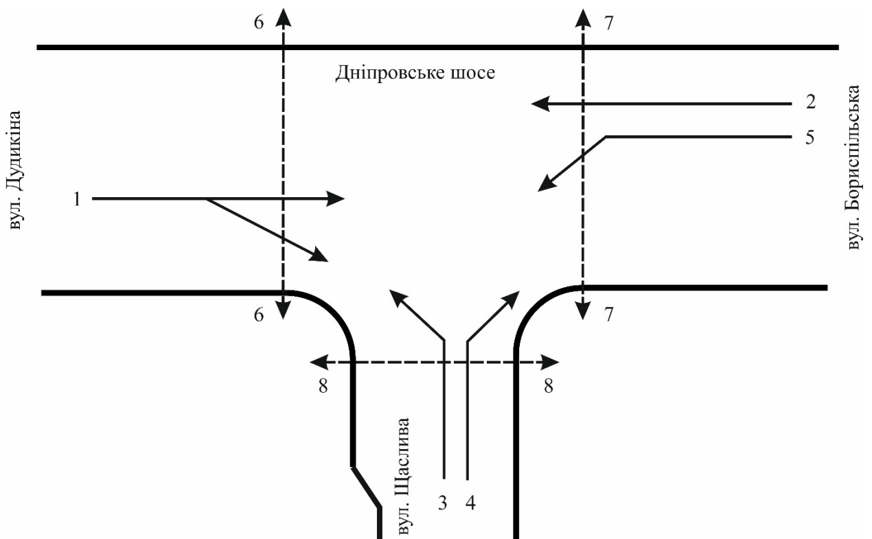
Рисунок 1.16 – Напрямки для дослідження об'ємів руху
