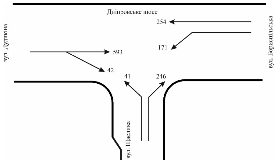
Рисунок 1.19 – Приведені об'єми руху (з 17:00 до 18:00)
