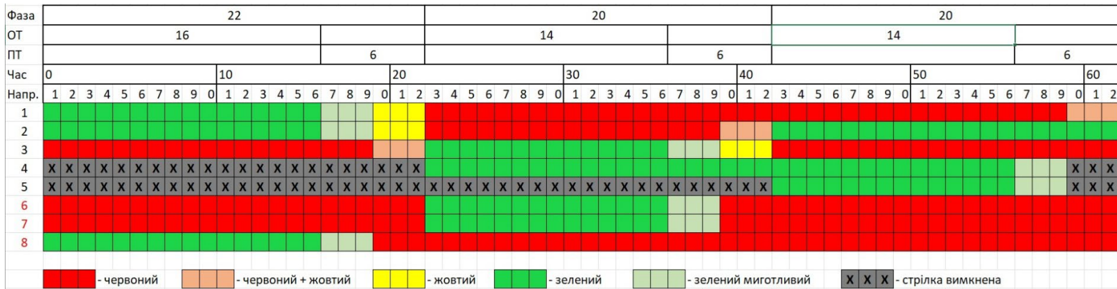
Рисунок 2.3 - Циклограма роботи світлофорів за програмою II
