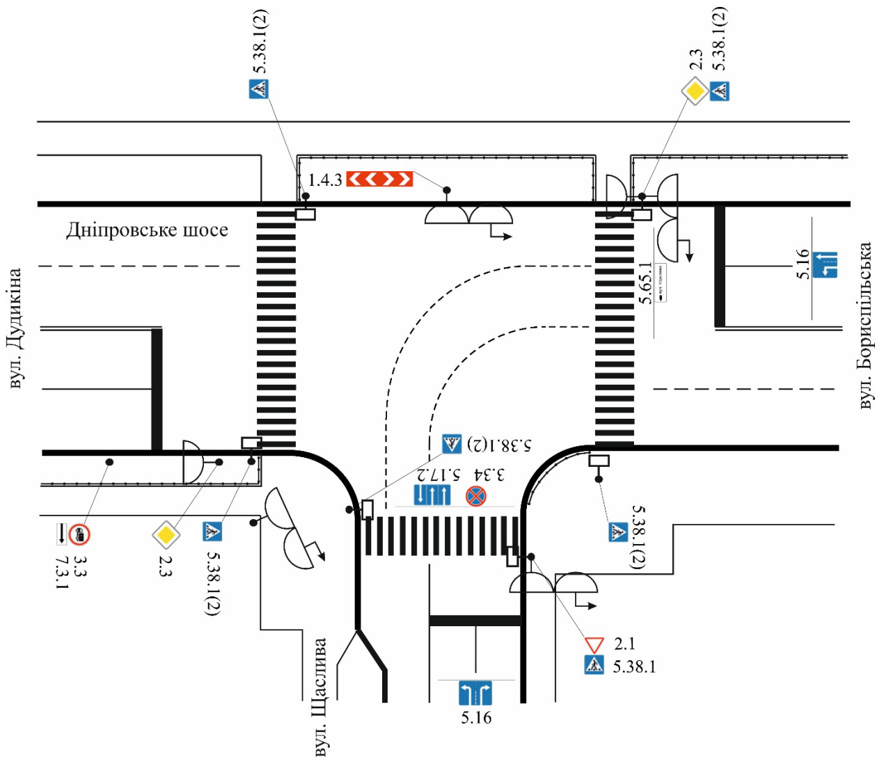
Рисунок 2.5 – Оновлена схема організації дорожнього руху на перехресті Дніпровського шосе із вулицею Щасливою
