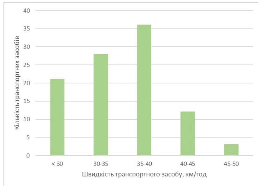
Рисунок 1.23 - Швидкості руху автомобілів вулицею Щасливою
