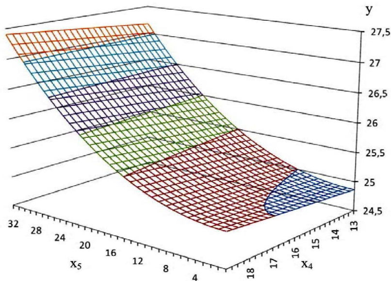
Рис. 4. Залежність загального зниження собівартості переділу виплавки сталі з використанням сплаву для легування та розкиснення ( y ) від вмісту у складі шихти суміші металевого порошку (шліфувального пилу силової обробки) сталі Р6М5 та Р6М5Ф3 ( x_4 ) та витрат феррохрому ( x_5 ), кг/т сталі
