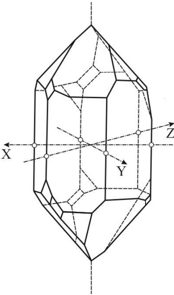
Рисунок 4.1 – Кристал кварцу \text{SiO}_2
