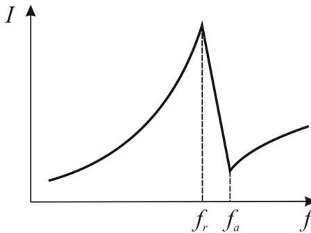
Рисунок 4.6 – Залежність сили струму в п'єзозразка від частоти
