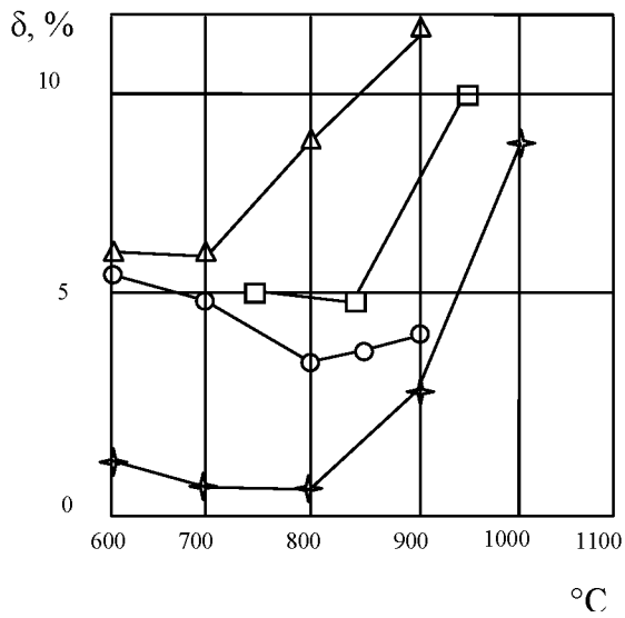
Рис. 2. Залежність \sigma_{0,2} , \sigma_{100} та ш ливарних термітних жароміцних сплавів на нікелевій основі від температури: ○ – для ЖСЗ; ✦ – для ЖС6; □ – для ВЖЗ6-Л1; △ – ВЖЛ8
