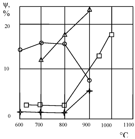
Рис. 2. Залежність \sigma_{0,2} , \sigma_{100} та ш ливарних термітних жароміцних сплавів на нікелевій основі від температури: ○ – для ЖСЗ; ✦ – для ЖС6; □ – для ВЖЗ6-Л1; △ – ВЖЛ8
