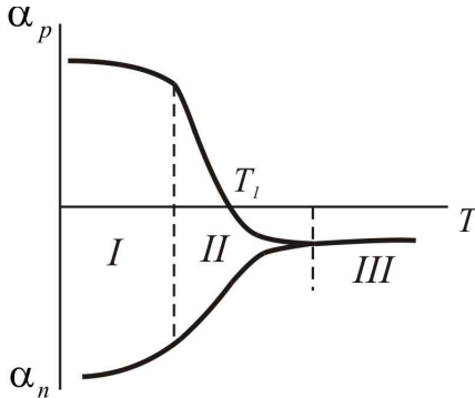
Рисунок 5.3 – Температурна залежність \alpha = f(T)
