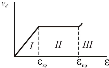
Рисунок 2.1 – Залежність дрейфової швидкості носія заряду v_d від напруженості електричного поля \mathcal{E} для кремнію і германію
