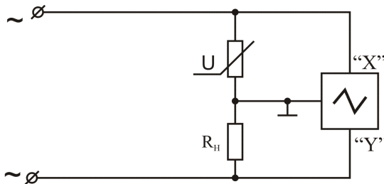
Рисунок 2.12 – Схема для дослідження ВАХ на змінному струмі
