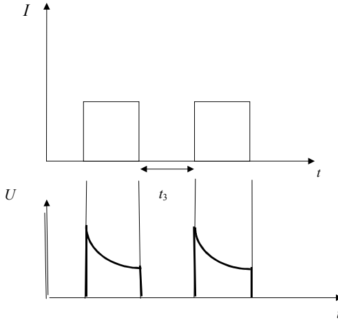
Рисунок 7.2 – Пара імпульсів струму (вгорі) і напруги (внизу)
