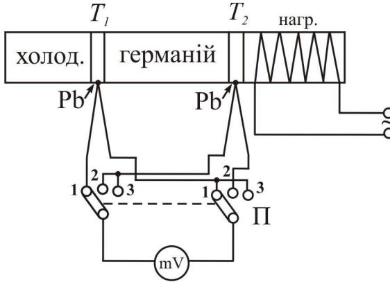
Рисунок 5.2 – Схема для зняття термо-ЕРС
