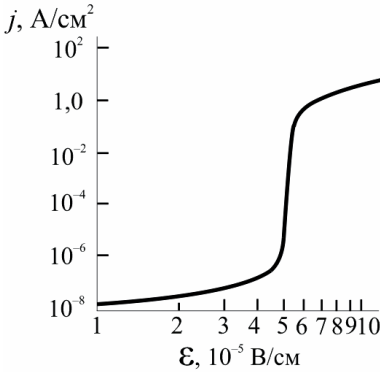
Рисунок 2.8 – Ударна йонізація в електронному германії за T = 4,2 \text{ K}
