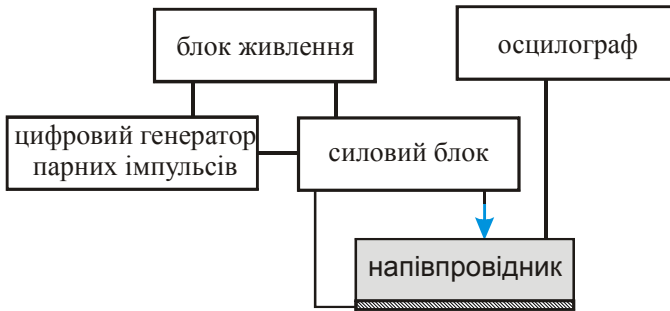
Рисунок 7.5 – Блок-схема модифікованої вимірювальної установки
