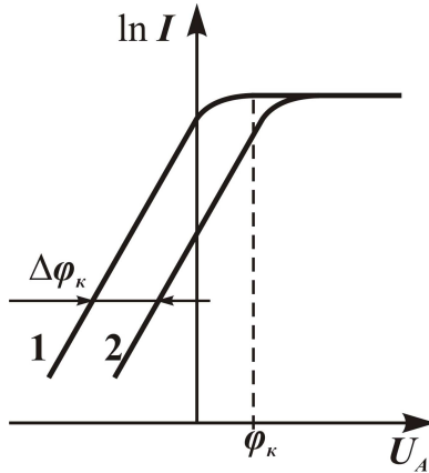
Рисунок 8.4 – ВАХ діода з напівпровідником в якості анода або катода
