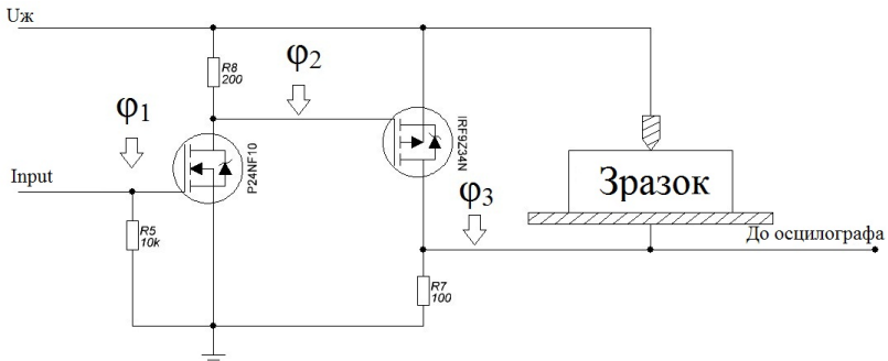
Рисунок 7.6 – Електрична принципова схема силового блоку
