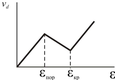
Рисунок 2.2 – Залежність дрейфової швидкості носія заряду v_d від напруженості електричного поля \mathcal{E} в арсеніді галію
