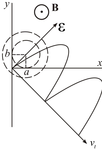
Рисунок 4.2 – Траєкторія руху електрона в схрещених електричному і магнітному полях
