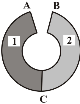
Рисунок 8.2. – Контакт двох різних металів
