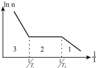
Рисунок 1.1 – Залежність концентрації електронів від температури донорного напівпровідника
