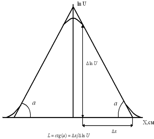
Рисунок 6.3 – Схема обчислення дифузійної довжини
