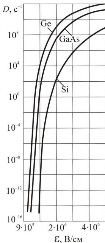
Рисунок 2.7 – Імовірність тунельного переходу електронів у залежності від напруженості електричного поля в p - n -переході
