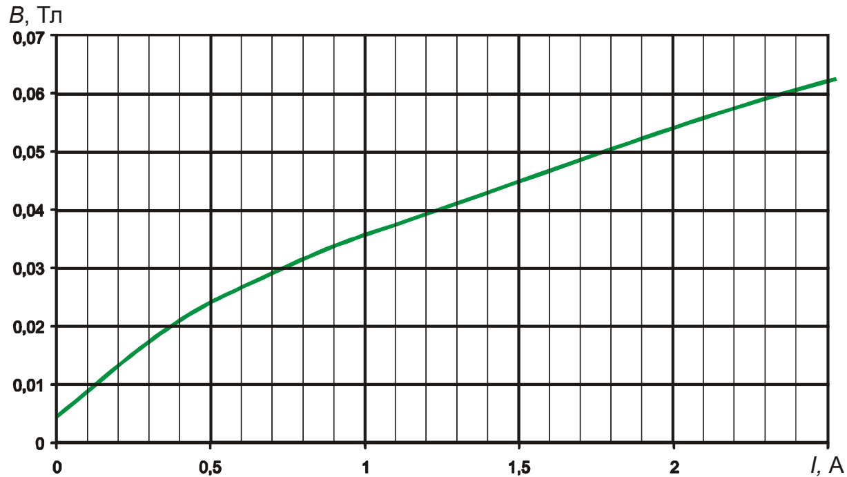
Рисунок В.1 – Графік залежності індукції магнітного поля від струму електромагніт
