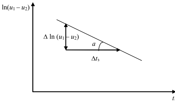
Рисунок 7.8 – Графік залежності \ln(\Delta U) від часу затримки імпульсу
