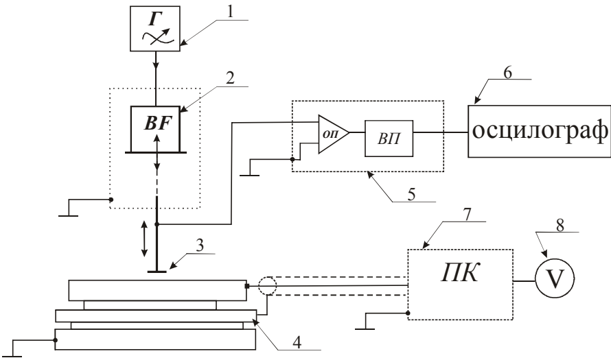
1 – генератор НЧ; 2 – перетворювач; 3 – електрод-еталон; 4 – столік; 5 – підсилювач; 6 – осцилограф; 7 – пристрій компенсації сигналу; 8 – вольтметр
