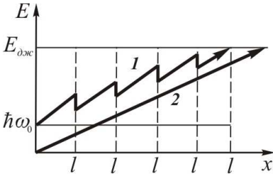
Рисунок 2.10 – Умовна діаграма ударної йонізації
