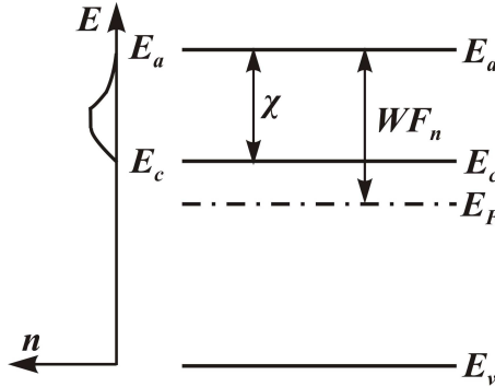
Рисунок 8.1 – Робота виходу електронів із напівпровідника
