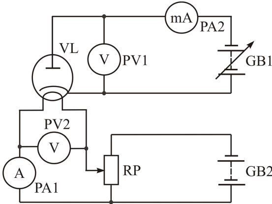
Рисунок 8.3 – Принципова схема для отримання ВАХ діода
