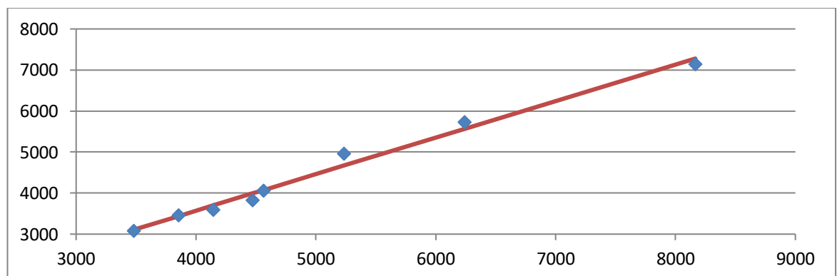
Рис. 3.1 Лінія регресії
