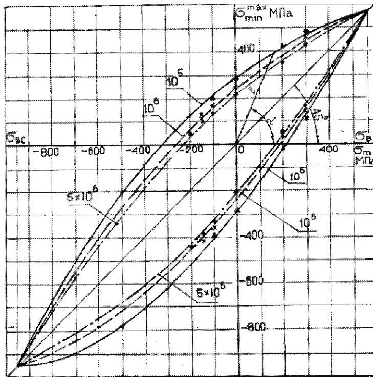
Рис. 5. Діаграма граничних напружень сталі 09Г2С
