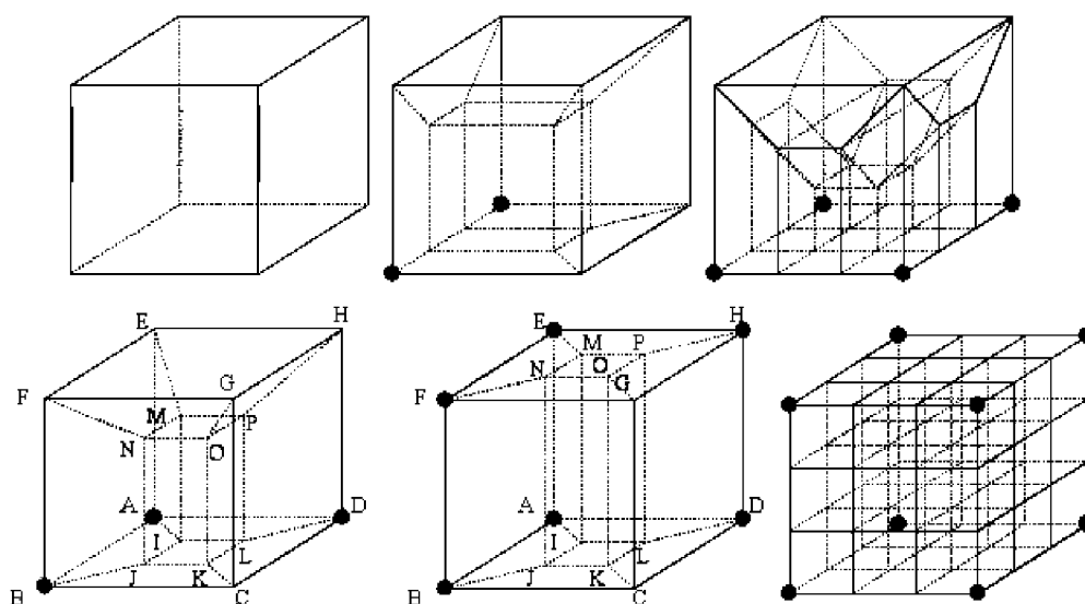
Рис. 9. Множество шаблонов 2
