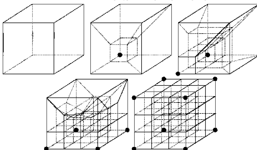
Рис. 7. Возможные конфигурации в трехмерном пространстве
