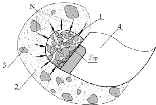
Рис. 4. Схема разрушения асфальтобетона баровым режущим инструментом: N – усилия, действующие на переднюю грань; 1 – уплотненное ядро; 2 – битумная связка; 3 – абразивные частицы; 4 – рабочая часть резца
