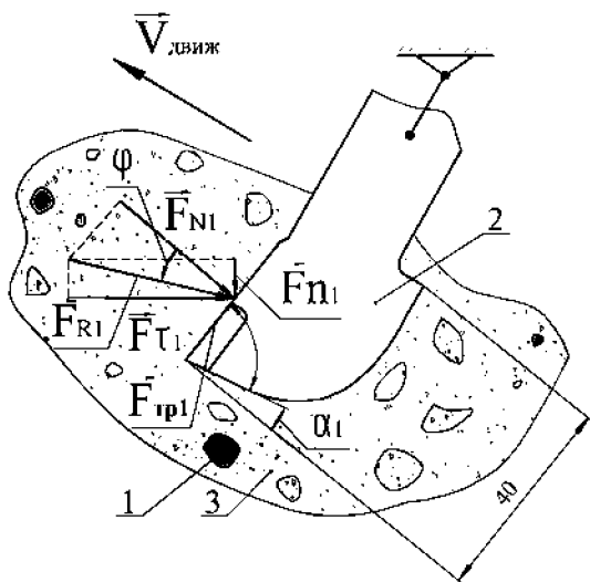
Рис. 1. Схема силового взаимодействия на переднюю грань реза бары при резании асфальтобетона: 1 – твердые частицы абразива; 2 – резец; 3 – битумная связка; F_{n1} – нормальная составляющая или сопротивление подачи реза на забой; F_{\tau1} – касательная составляющая или сопротивление резанию передней гранью реза; \alpha – угол резания инструмента; \varphi – угол трения грунта о сталь ( \varphi = 25...45^\circ ) [14]
