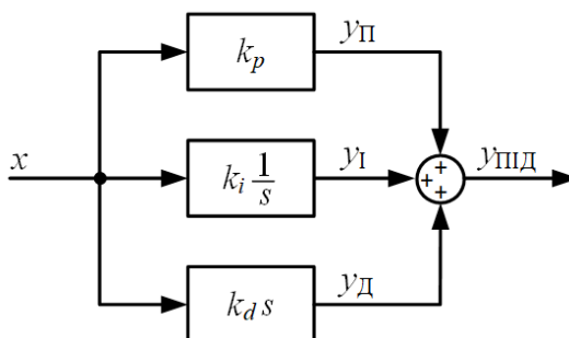
Рисунок 1.8 – Структурна схема ПД-регулятора
