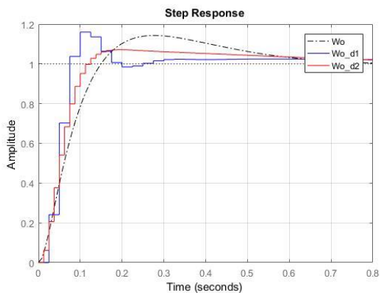
Рисунок 4.1 – Результати моделювання (за допомогою 'zoh')
