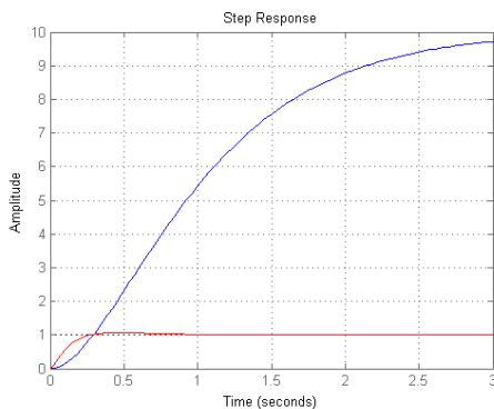
Рисунок 1.11 – Результати моделювання системи без ПІД та з ПІД-регулятором
