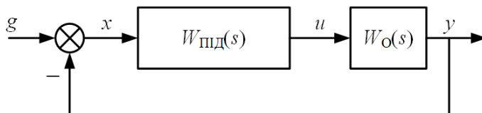
Рисунок 1.7 – Структурна схема САК з ПД-регулятором
