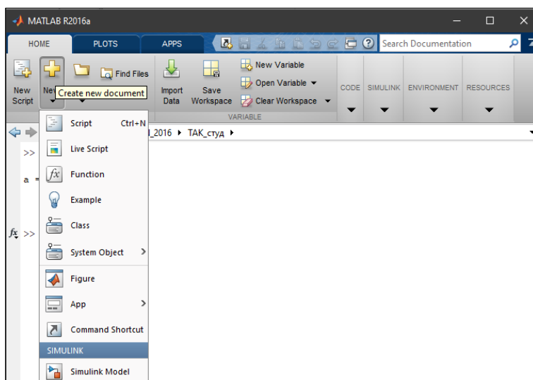
Рисунок 1.2 – Створення М-файлу
