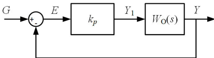
Рисунок 1.10 – Передатна функція ОК із Р-законом регулювання
