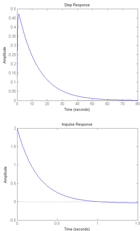
Рисунок 2.2 – Результати побудови часових характеристик для x_2
