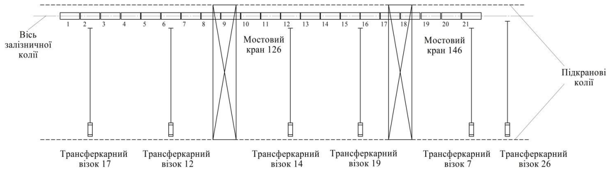
Рис. 1. Схема фронту відвантаження металопрокату
