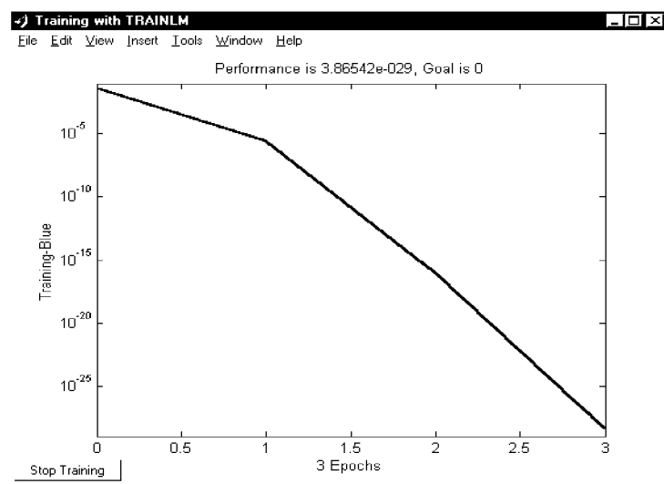
Рисунок 5.11 – Графік зміни значення цільової функції в процесі навчання
