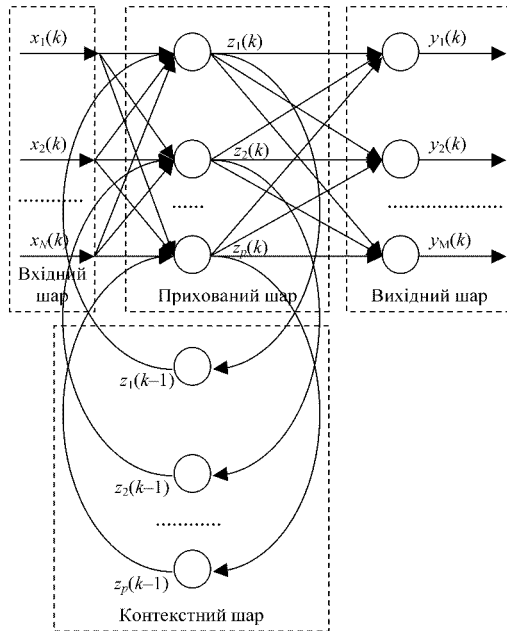
Рисунок 3.2 – Мережа Елмана
