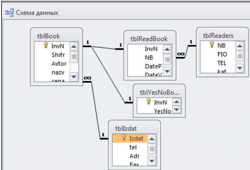
Рисунок 1.8 – Приклад схеми даних БД
