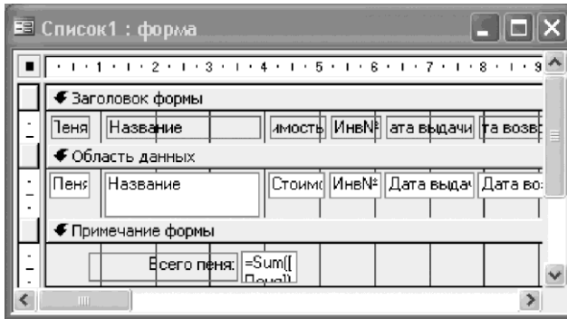
Рисунок 3.2 – Форма frmList1 в режиме конструктора
