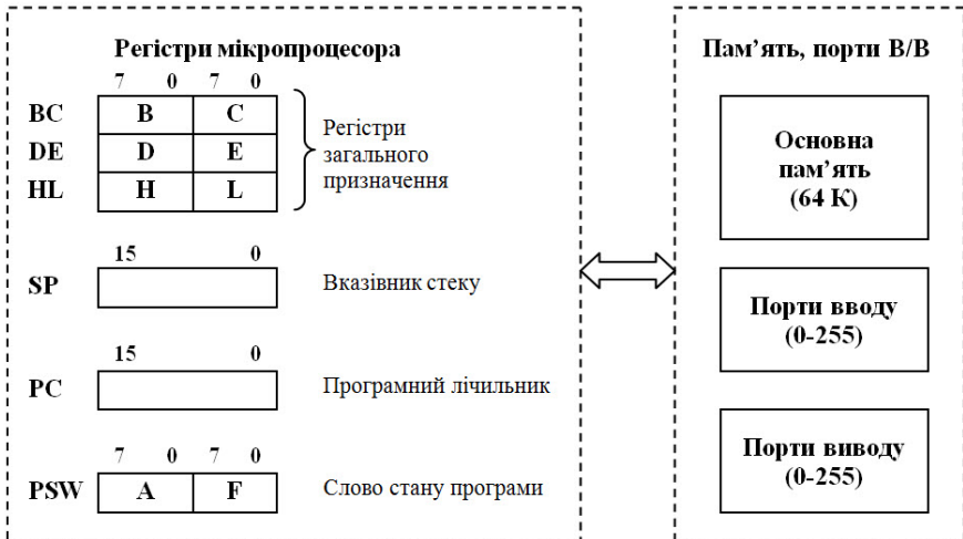
Рисунок А.1 – Програмістська модель МПС
