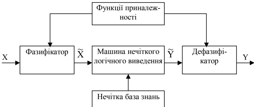
Рисунок Г.1 – Нечітке логічне виведення
