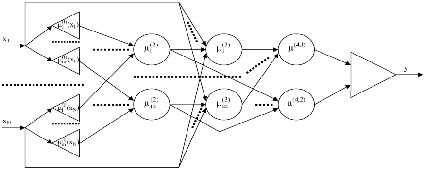
Рисунок В.2 – Мережа Такагі-Сугено-Канга
