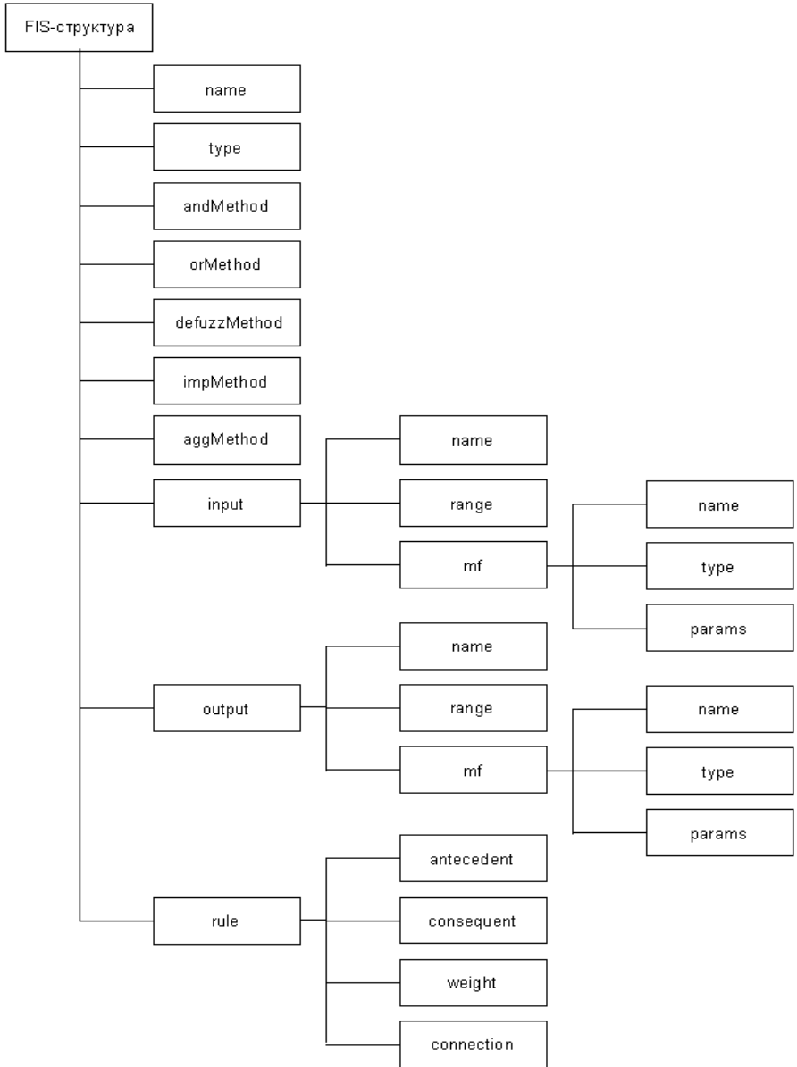
Рисунок Г.2 - FIS-структура
