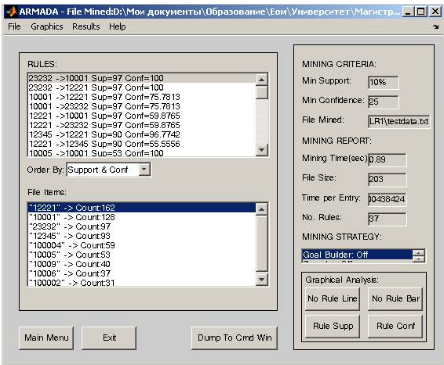
Рисунок А.2 – Результати аналізу даних за допомогою модулю ARMADA
