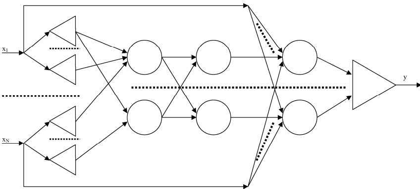
Рисунок В.3 – Мережа ANFIS
