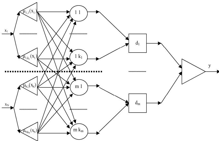
Рисунок В.1 – Структура нейро-нечіткої мережі Мамдані
