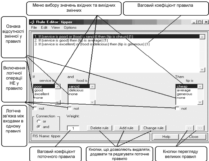
Рисунок Г.5 - Редактор бази знань
