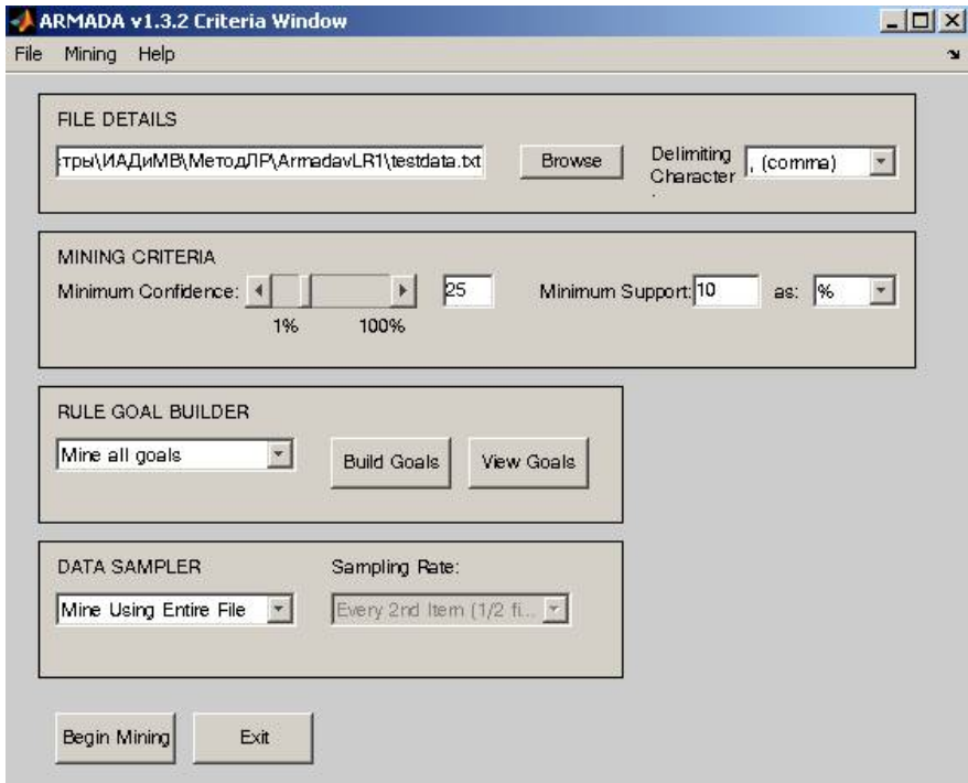
Рисунок А.1 – Головна інтерфейсна форма модулю ARMADA
