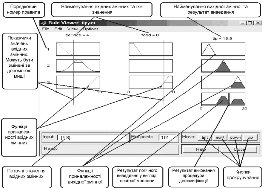
Рисунок Г.6 – Візуалізація логічного виведення для системи tipper за допомогою Rule Viewer
