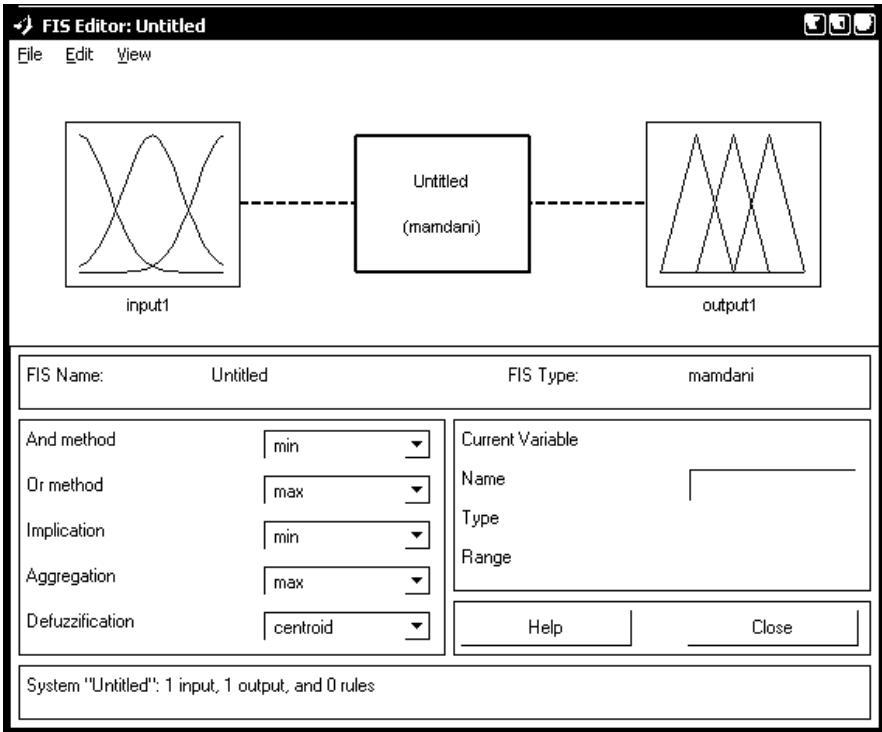
Рисунок Г.3 - FIS-редактор
