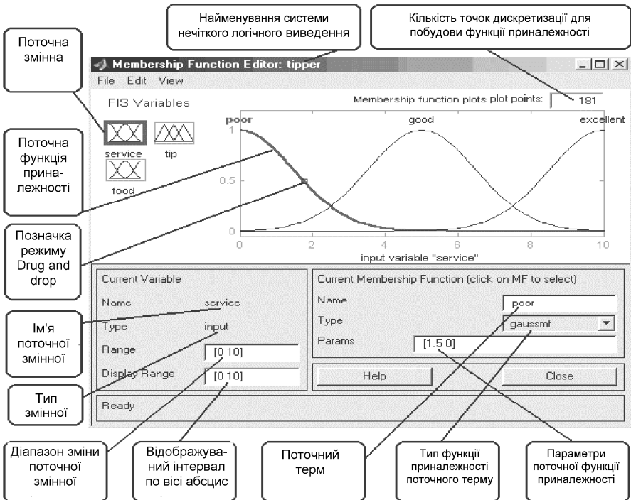
Рисунок Г.4 - Редактор функцій приналежності
