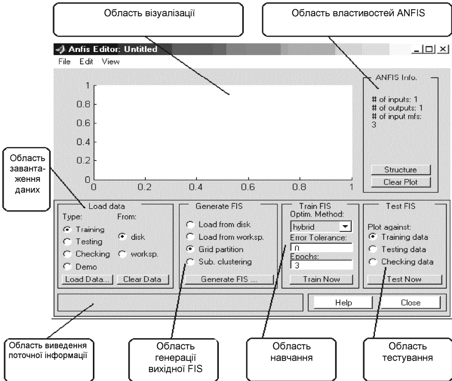
Рисунок Г.7 - Основне вікно ANFIS-редактора
