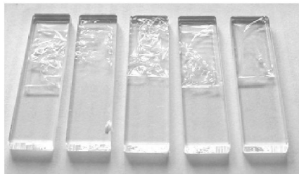
Рис. 3. Руйнування у вакуумній камері незахищених частин поверхні пластин з оптичного скла К8 після їх електронно-променевої обробки в оптимальному режимі ( P_{\text{min}} = 2 \cdot 10^2 \text{ Вт/см}^2 , T_0 = 510 \text{ }^\circ\text{C} , V_{\text{ном}} = 2,7 \text{ см/с} ) потоку та подальшого прискореного охолодження ( V_{\text{охол}} \geq 10 \text{ }^\circ\text{C/с} )
