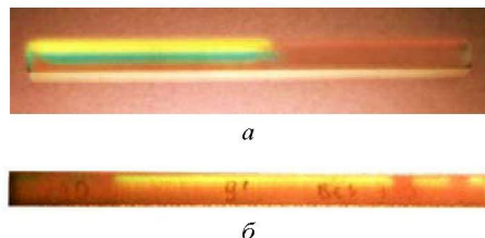
Рис. 5. Картина подвійного променезаломлення у прямокутних пластинах зі скла К8, поверхня яких оброблена електронним потоком через з'ємну маску Ні (а) та через напилену тонку плівку Ні (б). Час охолодження 12 годин
