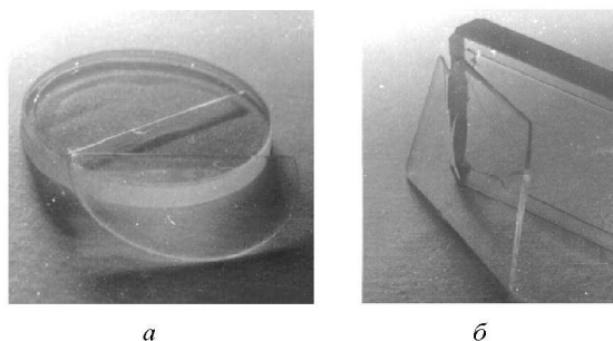
Рис. 6. Відшаровані ПШ від пластин різної форми зі скла К8 після електронно-променевої мікрообробки: а – кругла пластина діаметром 20 мм, товщиною 4 мм; б – прямокутна пластина 70 \times 14 \times 4 \text{ мм}
