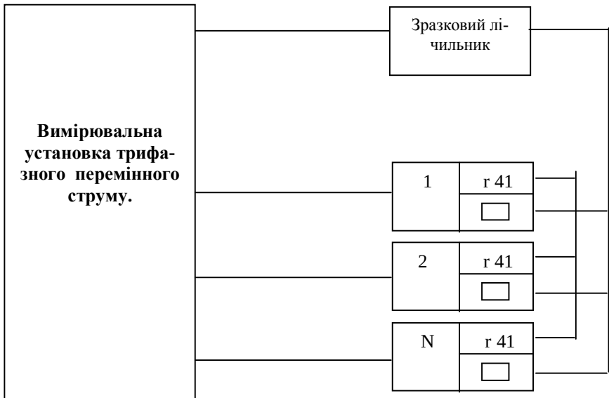
Рисунок 2.6 – Структурна схема перевірки лічильника сімейства ZU і ZB методом зразкового лічильника
