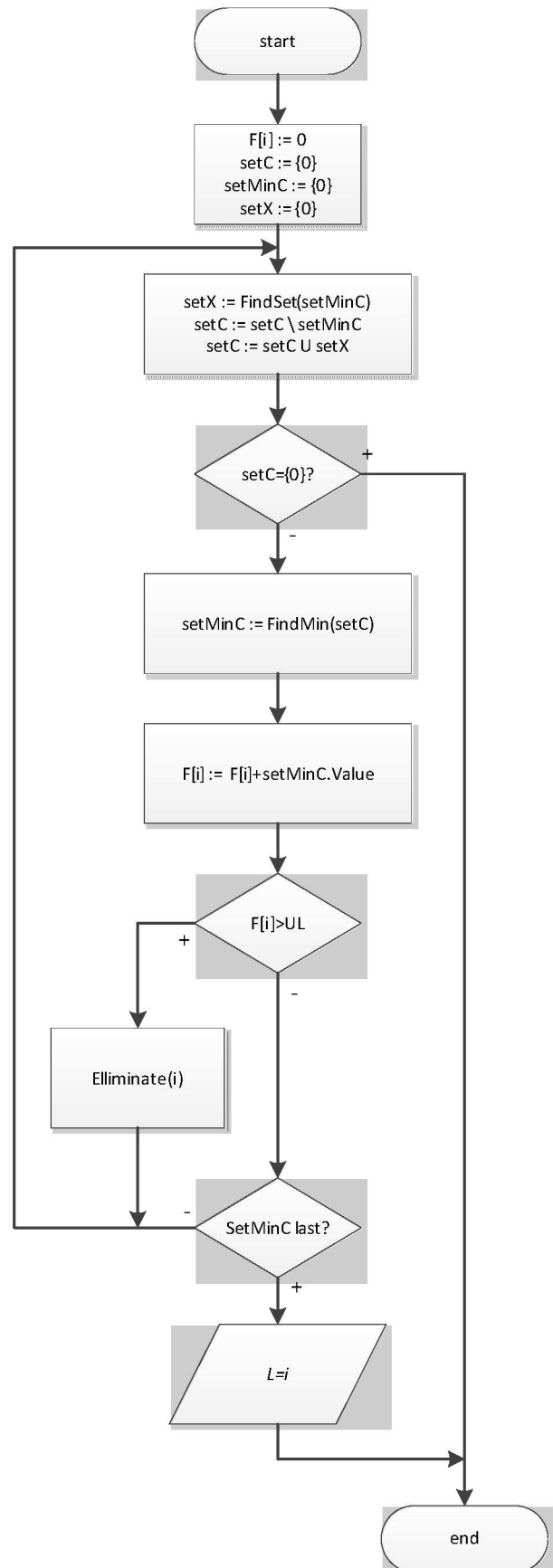
Рис. 3. Граф-схема алгоритма
