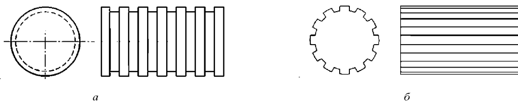
Рис. 1. Валки с поперечными (а) и продольными (б) проточками
