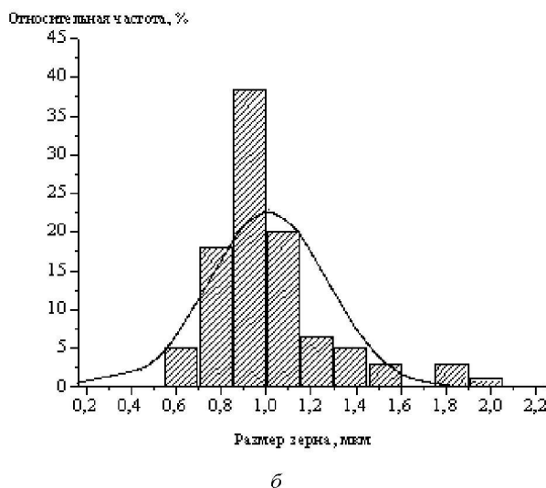
Рис. 6. Типичное изображение структуры, полученной после прокатки по режиму № 4 ( a ) и ее частотное распределение по размерам зерен ( б ), a – оптическая микроскопия, \times 500
