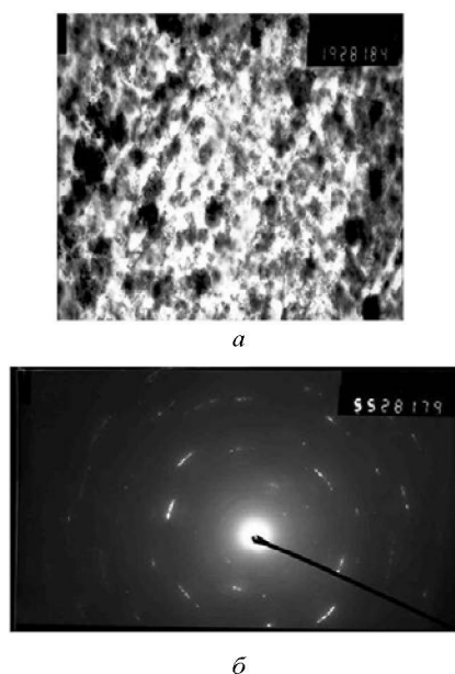
Рис. 5. Микроструктура меди после прокатки со сдвигом по режиму № 4:
