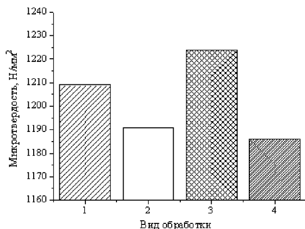
Рис. 8. Изменение микротвердости образца в зависимости от способа прокатки:
