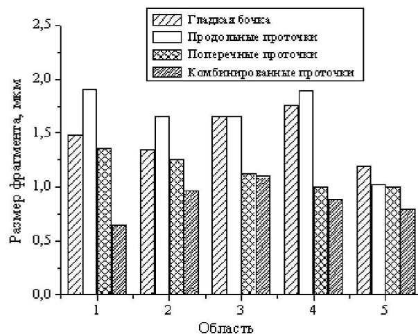
Рис. 4. Зависимость размера фрагмента от места вырезки образца для разных видов прокатки
