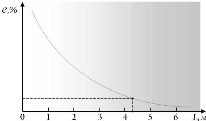
Рисунок 6.1 - Графік зміни КПО у приміщенні
