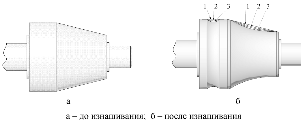
Рисунок 1 – Схема изнашивания рабочей поверхности бочки вала
