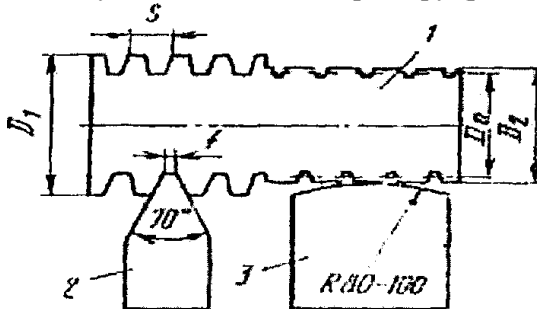
Рисунок 2.2 - Схема електромеханічної висадки та
