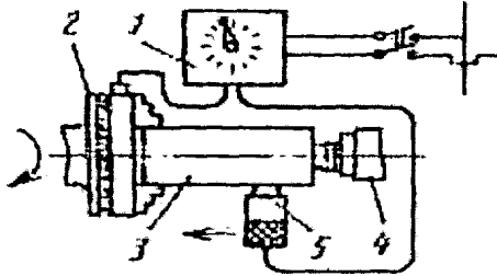
Рисунок 2.1 - Схема електромеханічної обробки
