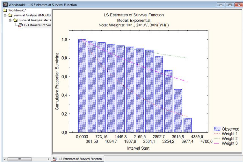
Рисунок 6.5 – Функція надійності
