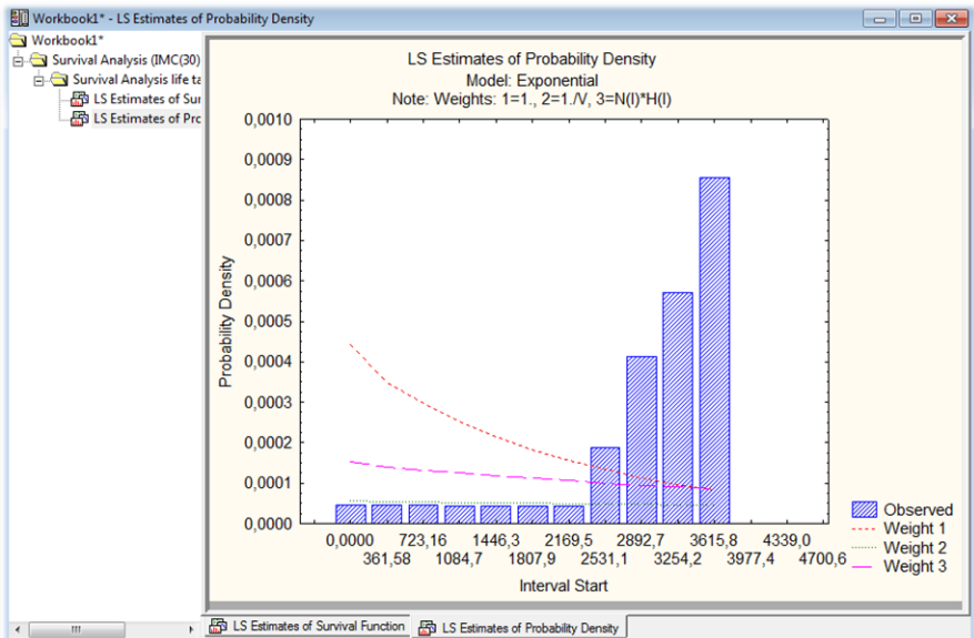
Рисунок 6.6 – Густина (щільність) функції надійності
