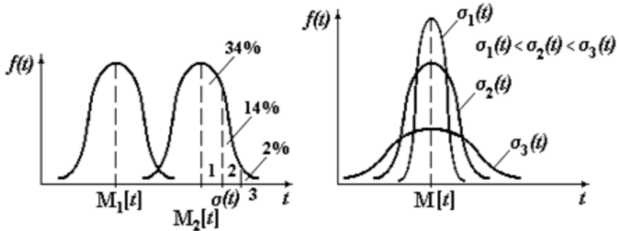
Рисунок 2.1 – Густина ймовірності при нормальному законі розподілу
