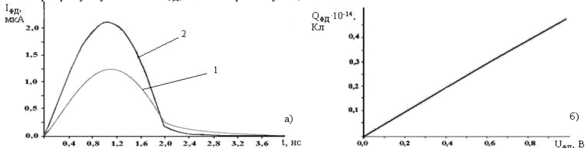
Рис. 7 - Частина результатів розрахунків параметрів ІК р-і-п ФД
