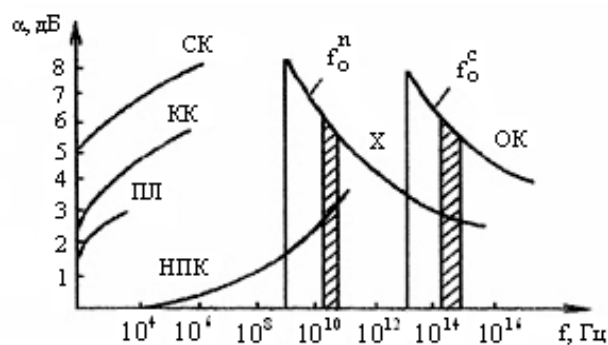
Рис. 2 - Частотні залежності загасання напрямних середовищ: КК – коаксіальний кабель, СК – симетричний кабель, ПЛ – повітряна лінія, НПК – надпровідний кабель, ОК – оптичний канал (кабель), X – хвилевід
