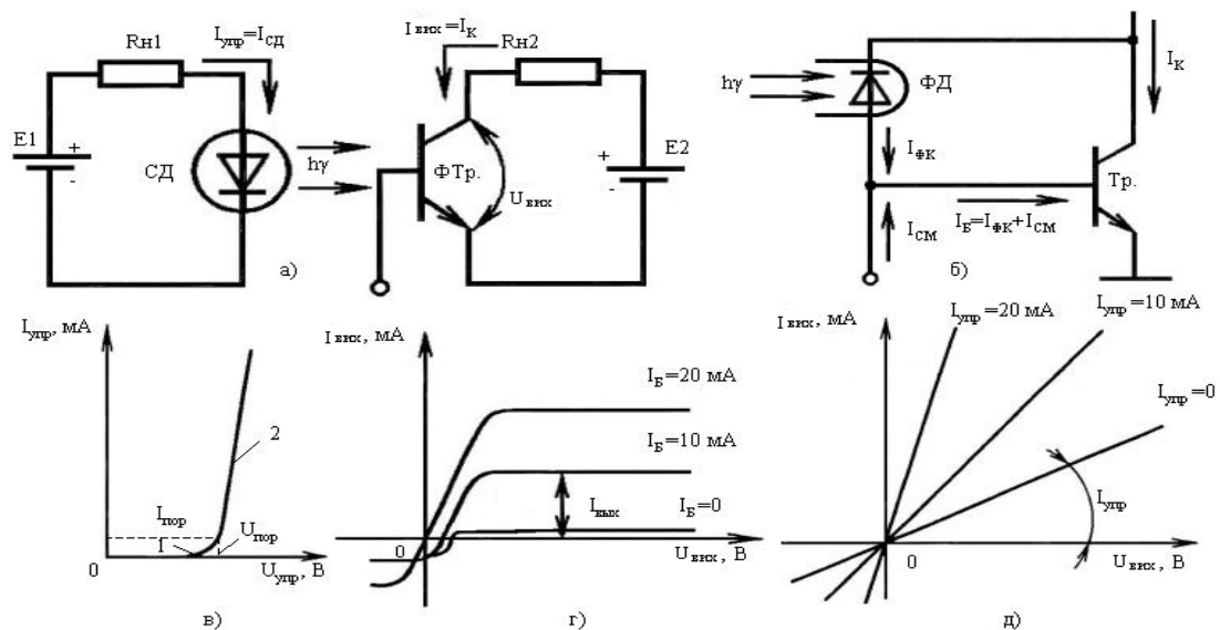
Рис.5 - Електрична схема ОЕП і його ВАХ: а – схема включення фототранзисторної оптопари (СД-ФТр); б – еквівалентна схема p-р-п фототранзистора; в – вхідна характеристика оптопари (ВАХ СД); г – характеристика фототранзисторної оптопари по виходу; д – характеристика фоторезисторної оптопари (СД-ФР) по виходу
