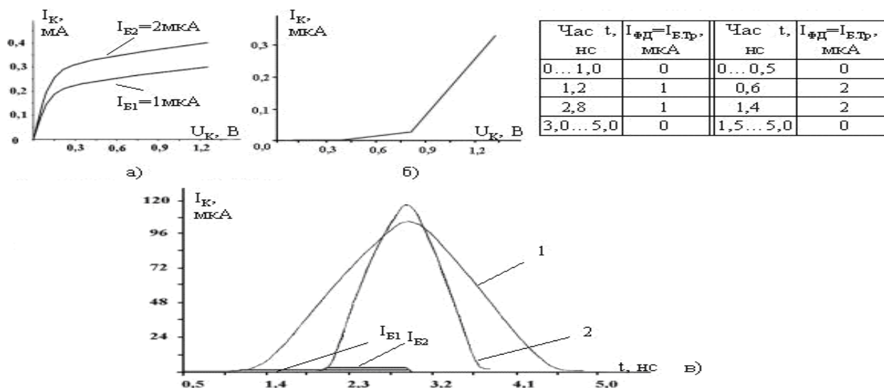
Рис. 8 - Частина результатів розрахунків параметрів інтегрального ВЧ п-р-п Тр
