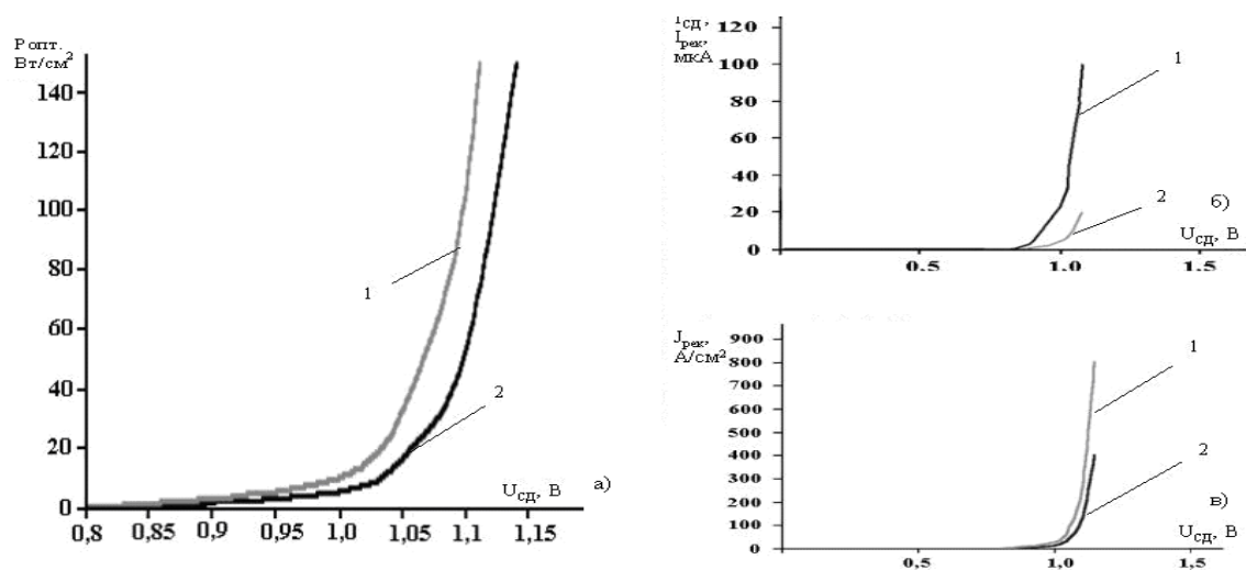
Рис. 6 - Частина результатів розрахунків параметрів мікропотужного ІК СД
