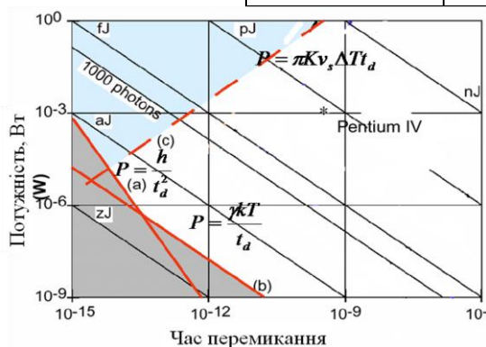
Рис. 1 - Графік досягнутих середніх значень параметрів логічних вентилів (біле поле праворуч): потужності ( P_{\text{вик.сер.}} , Вт), часу ( t_{\text{зт.сер.}} , нс) і роботи перемикання ( A_{\text{сер.}} , пДж) та обмеження властивостей НП матеріалів для Si (сіре поле); * - параметри Pentium IV
