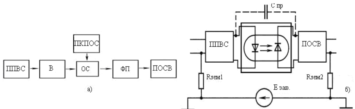
Рис. 3 - Узагальнена функціональна схема оптоелектронного пристрою – а; схема оптоелектронного каналу з урахуванням протікання струмів завад крізь паразитні зв'язки – б; ППВС – пристрій перетворення вхідного сигналу, В – випромінювач, ПКПОС – пристрій керування параметрами оптичного середовища, ОС – оптичне середовище, ФП – фотоприймач, ПОСВ – пристрій обробки сигналу на виході, Е зав. – ЕДС наведеної завади
