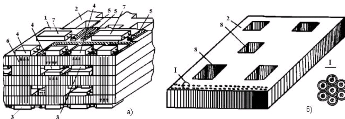
Рис. 4 - Реалізація оптичних міжблочних зв'язків на основі пристроїв типу волоконно-оптична пластина (ВОП): а - конструкція у зборі; б - ВОП із ВОК: 1 - плата; 2 - ВОП з ВОК; 3 - блок світлодіодів; 4 - блок ФП; 5 - струмопровідні доріжки; 6 - хід оптичних променів; 7 - мікросхема; 8 - вікна для електричних зв'язків; І - збільшений вид зверху на ВОК, що складають ВОП
